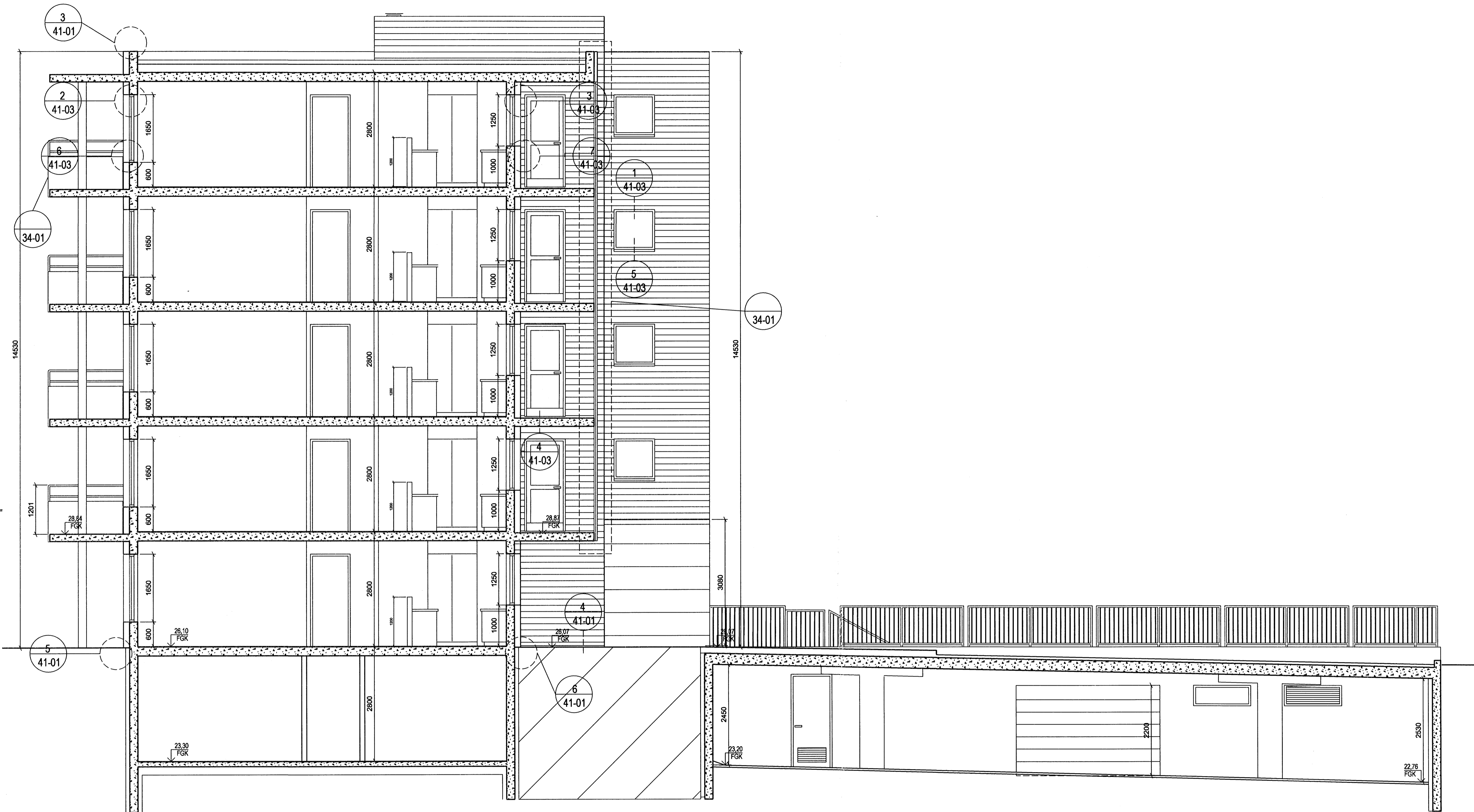
SNID A-A 1:50
