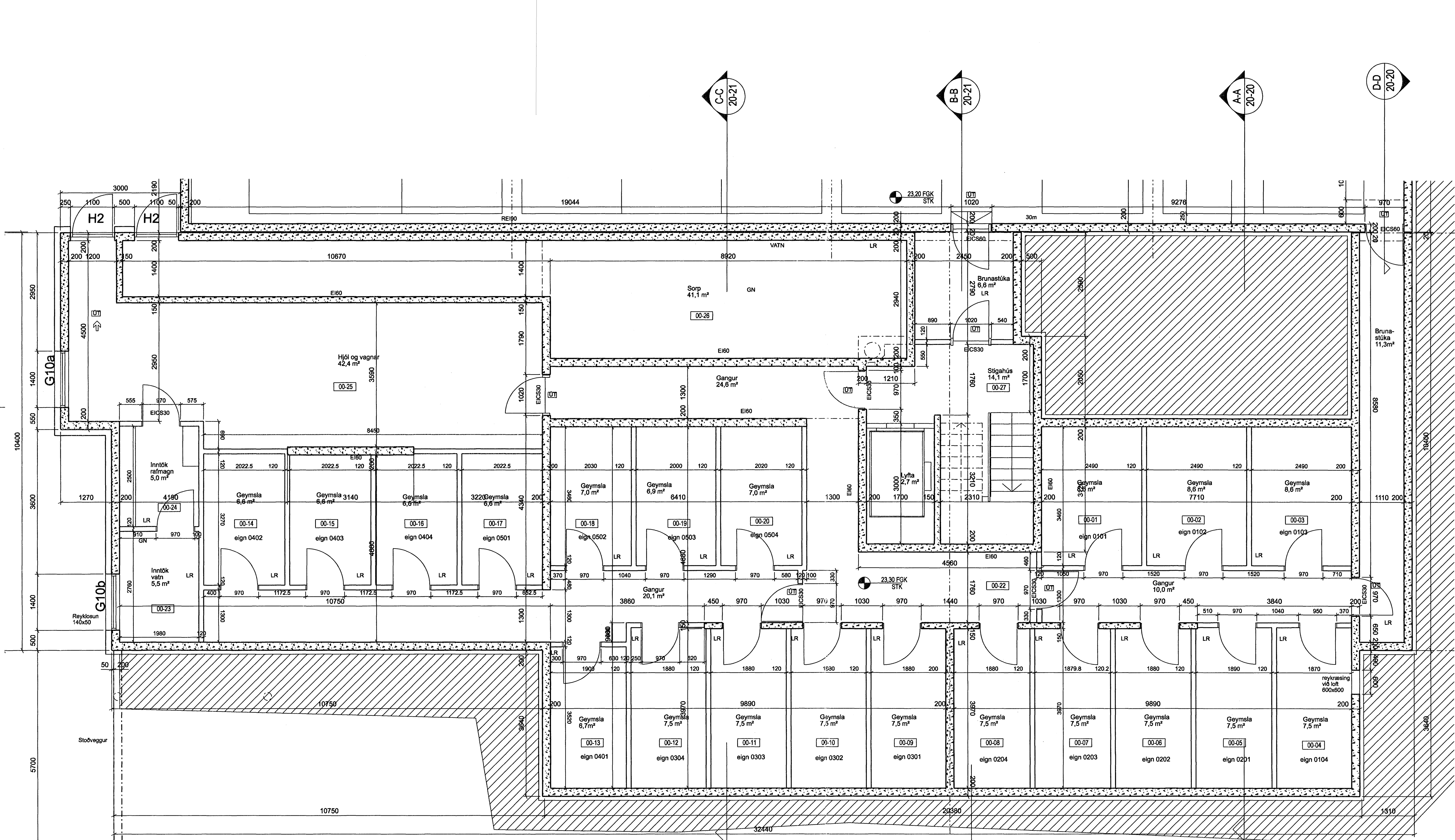
GRUNNMYND 1:50 Kjallari
