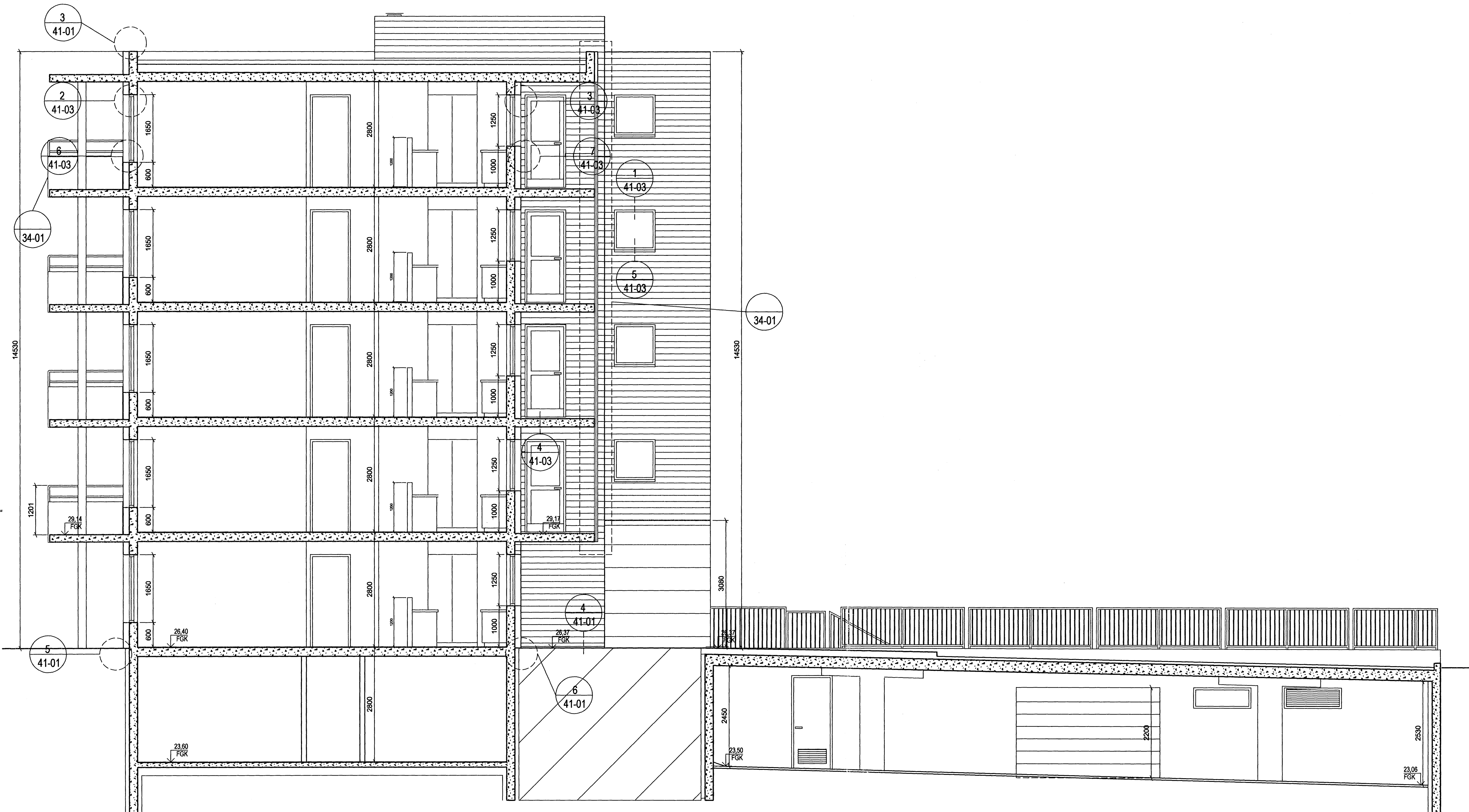
SNID A-A 1:50
