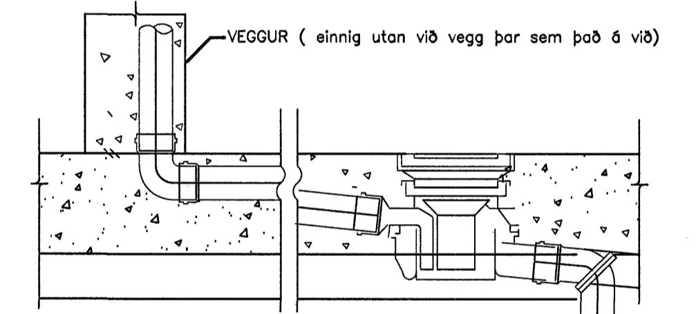
GÓLFENDURFALL MED GEGNUMRENNSLI, 1:5
