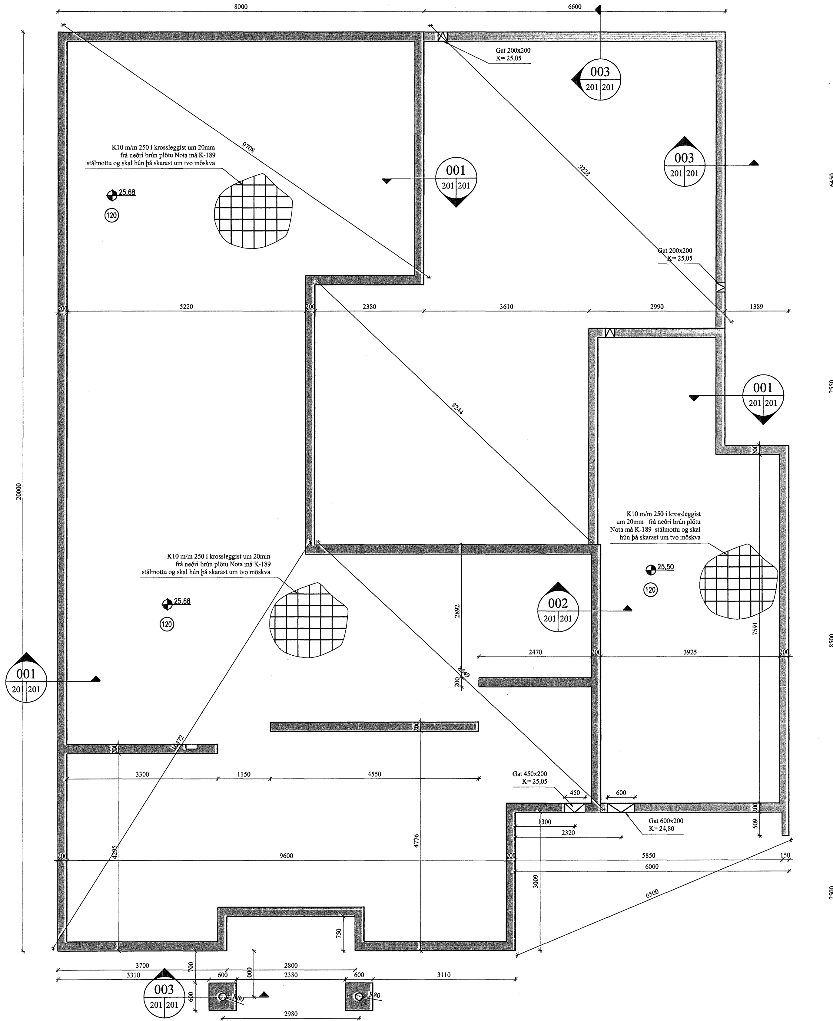
GRUNNMYND SÖKKLA OG PLÖTU Mkv: 1/50
