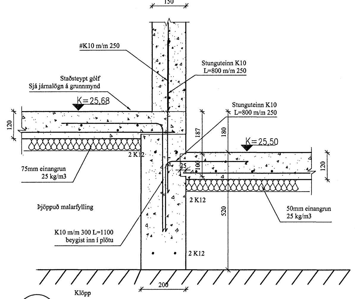
002 SKURÐUR Í SÖKKULÚRTVEGG 201|201 Mkv: 1/10
