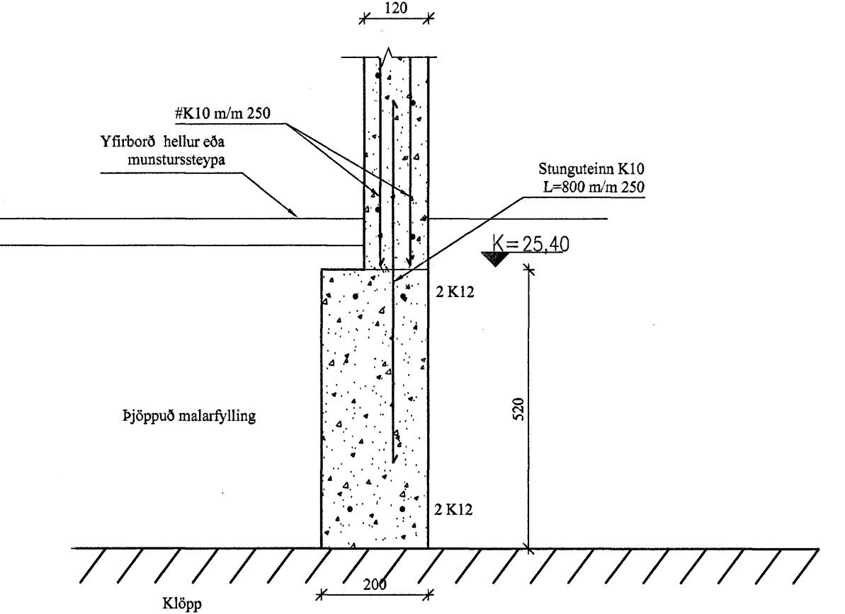
003 SKURÐUR Í SÖKKULÚRTVEGG 201|201 Mkv: 1/10
