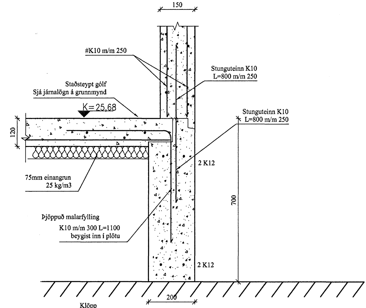
001 SKURÐUR Í SÖKKULÚRTVEGG 201|201 Mkv: 1/10
