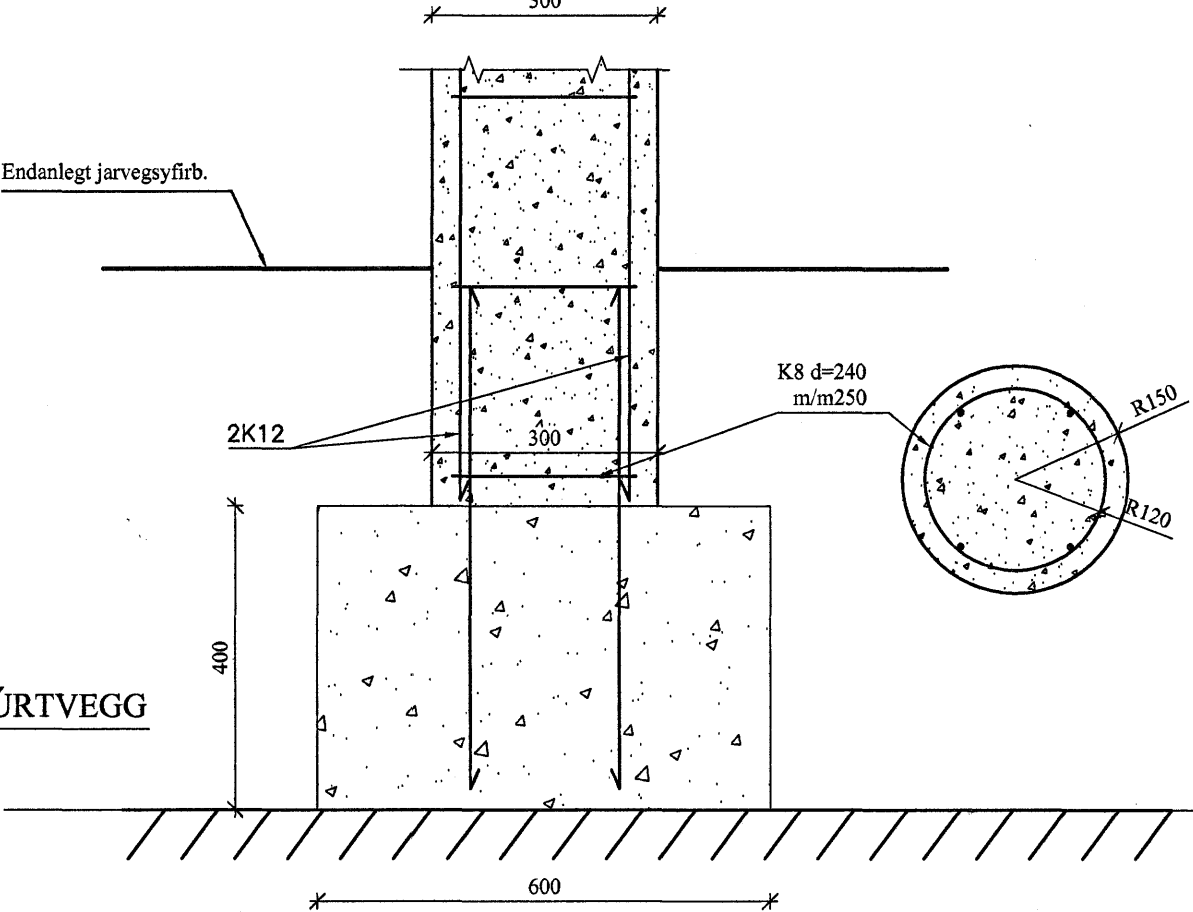
003 SKURÐUR Í SÖKKULÚRTVEGG 201|201 Mkv: 1/10
