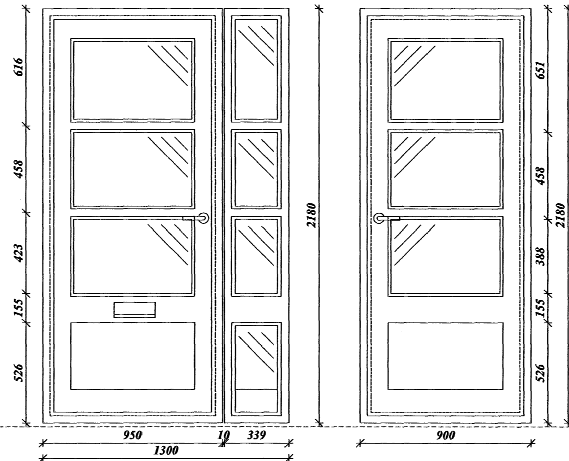
Hurð gerð A opnun inn til hægri Fjöldi 1 stk.
