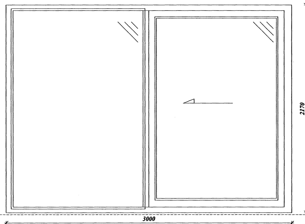
Hurð með rennihurð gerð D (stellið er út úr elúhústi að verönd) Fjöldi 1 stk.
