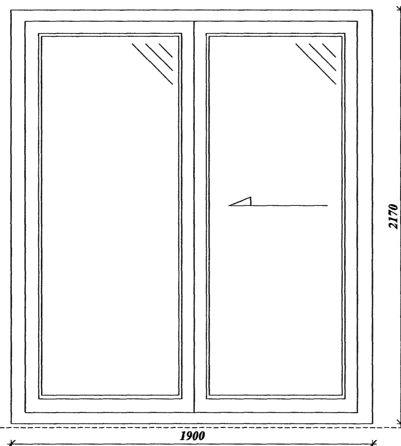
Hurð með rennihurð gerð C (stellið er út úr sjónvoppsstofu) Fjöldi 1 stk.
