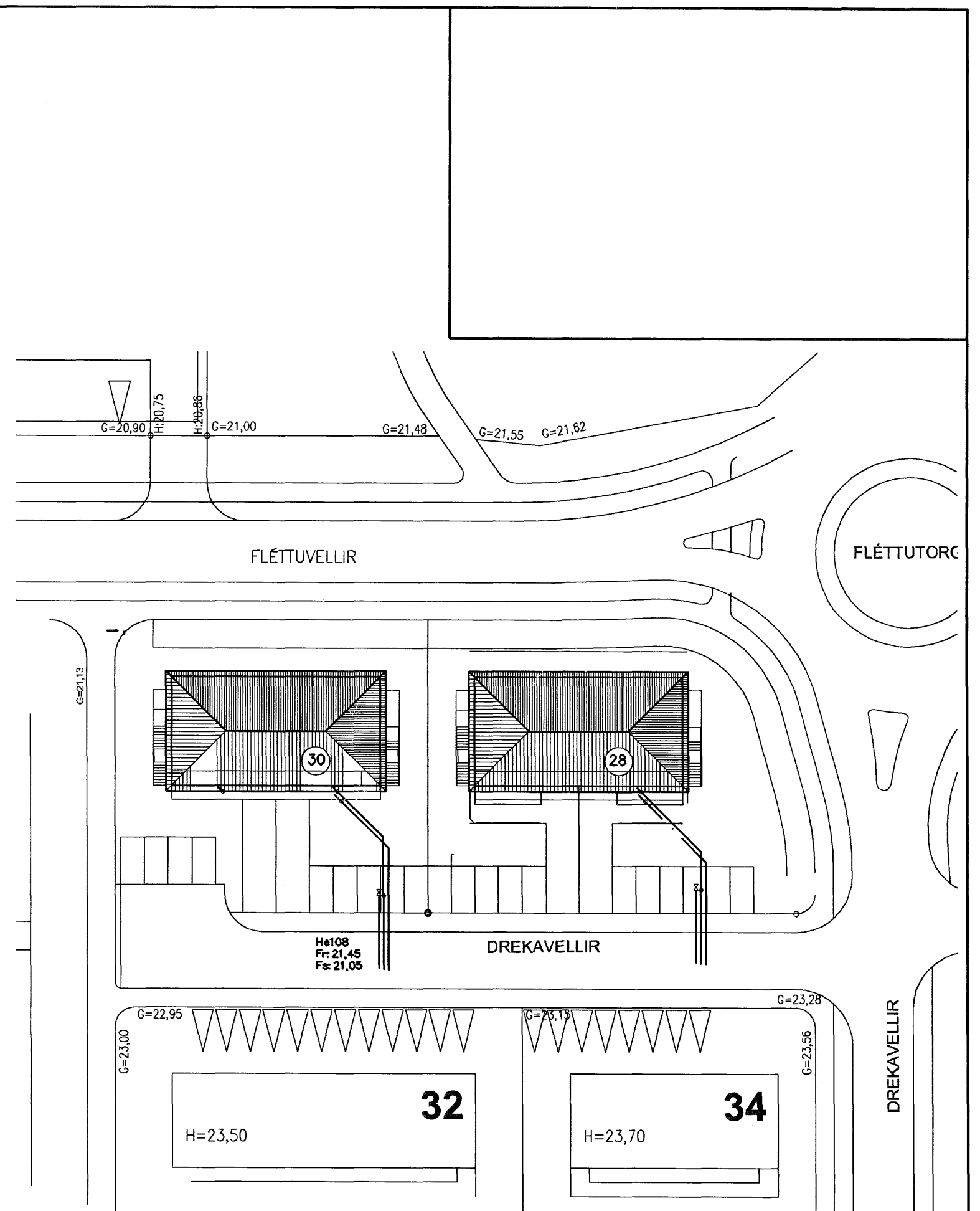
Afstöðmynd, 1:500
