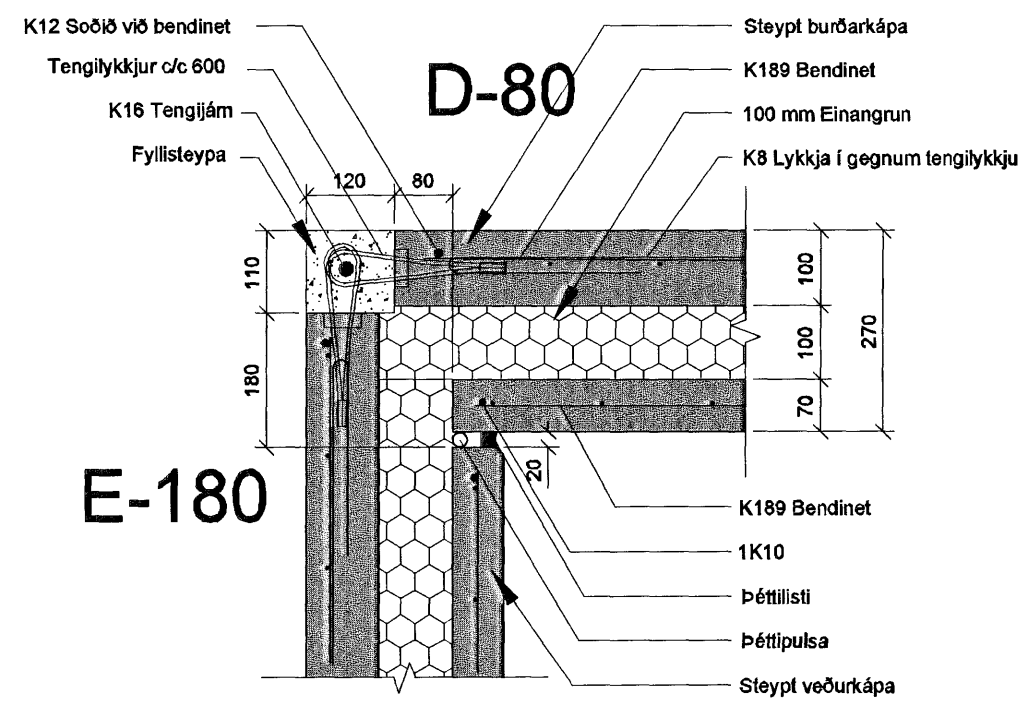
B-104 - Innhorn SNIÐ. 1:10
