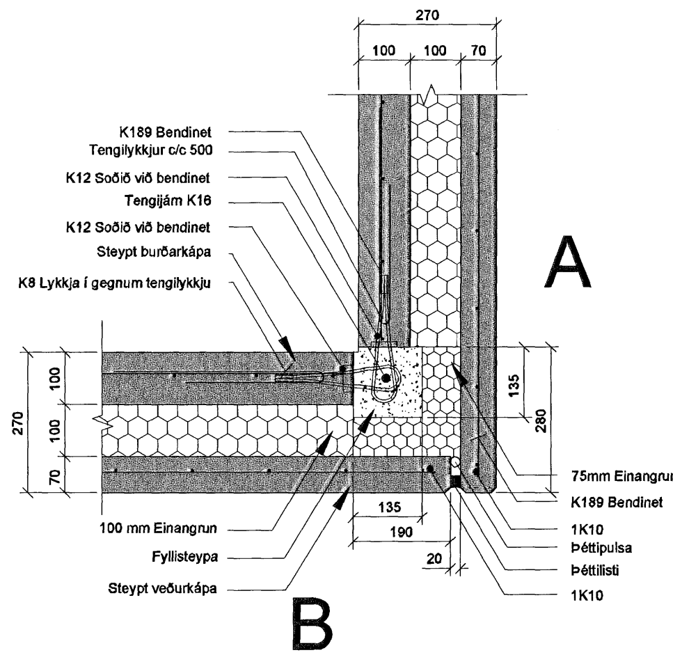
A-104 - úthorn SNIÐ. 1:10
