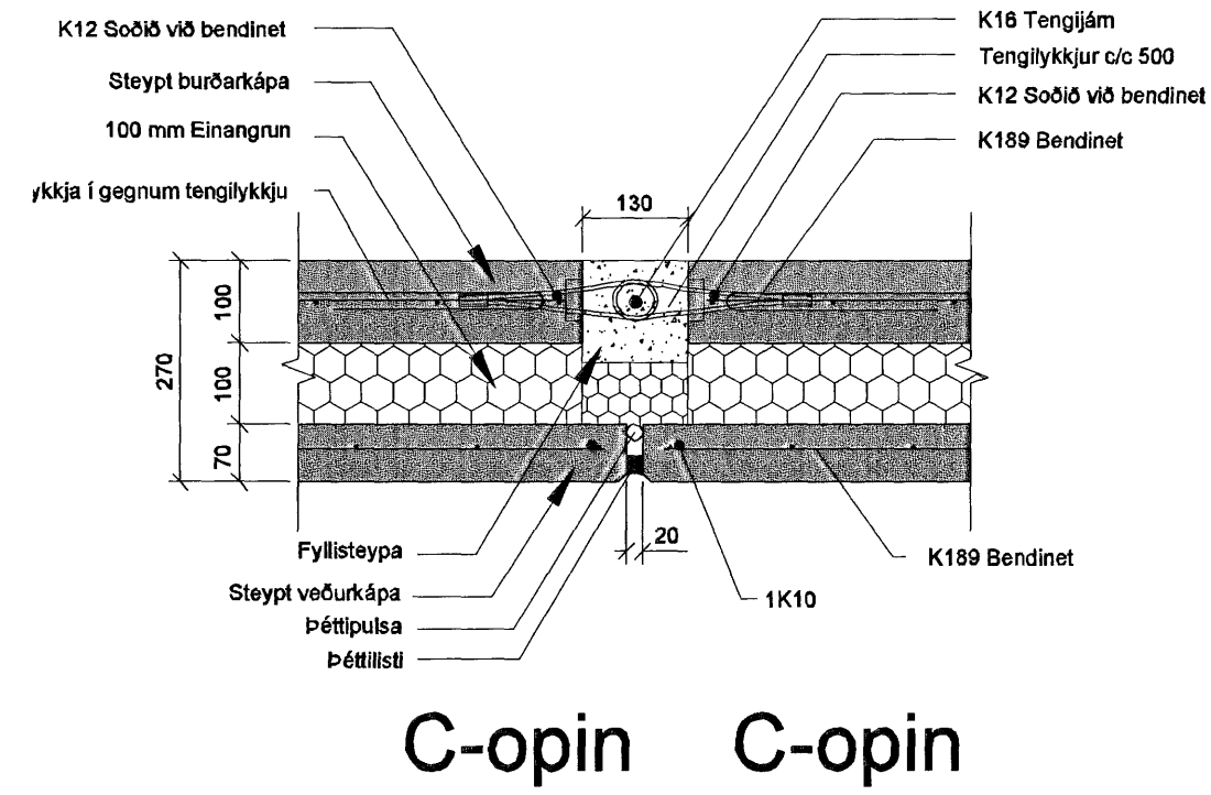
C-104 - samsetning SNIÐ. 1:10
