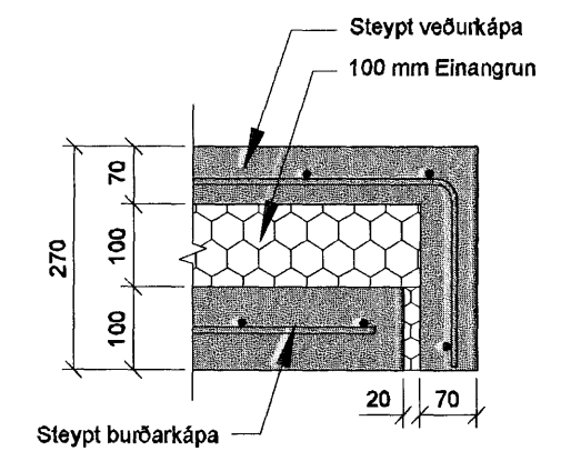
G-104 SNIÐ. 1:10
