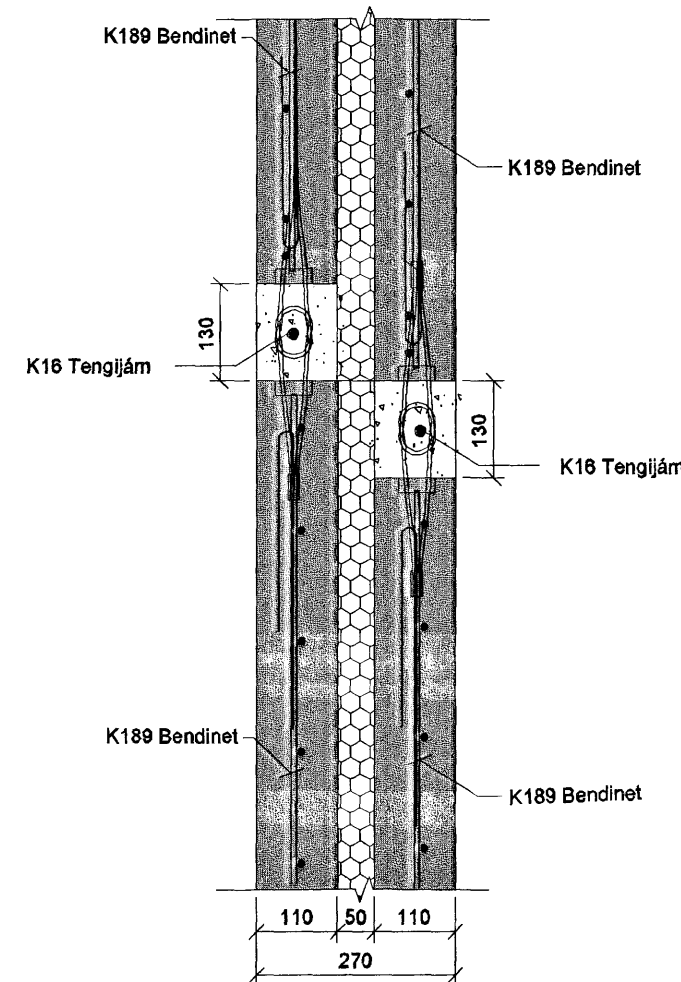
F-104 SNIÐ. 1:10
