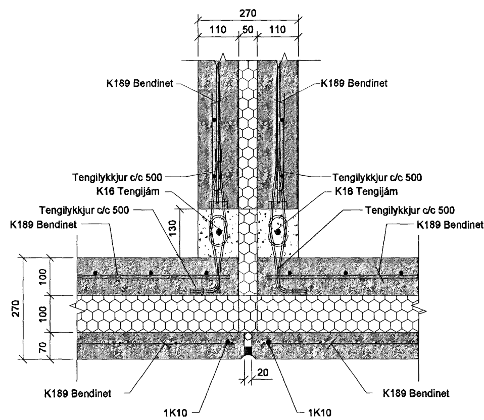
D-104 SNIÐ. 1:10
