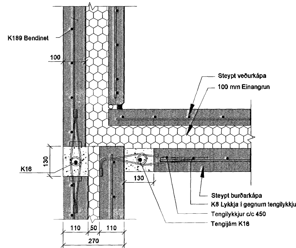
E-104 SNIÐ. 1:10
