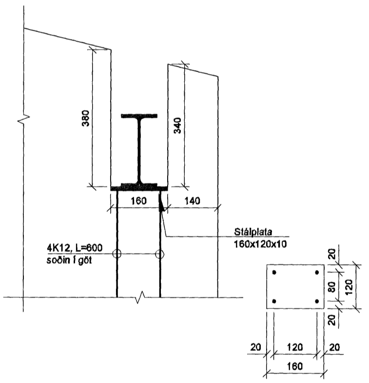
E-107 SNIÐ. 1:10
