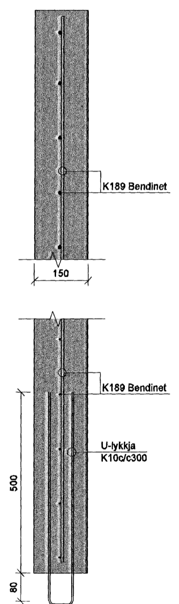
B-107 SNIÐ. 1:10
