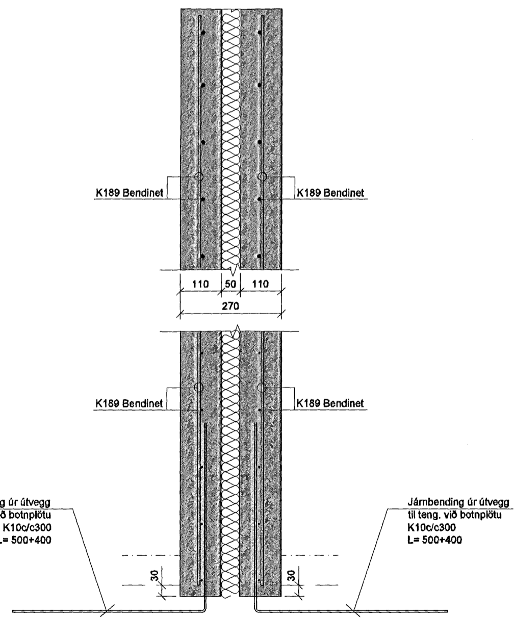
A-107 SNIÐ. 1:10
