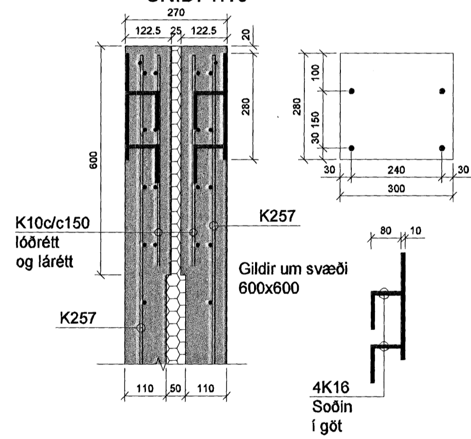
D-107 SNIÐ. 1:10
