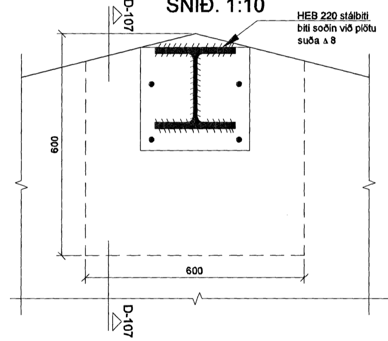
C-107 SNIÐ. 1:10
