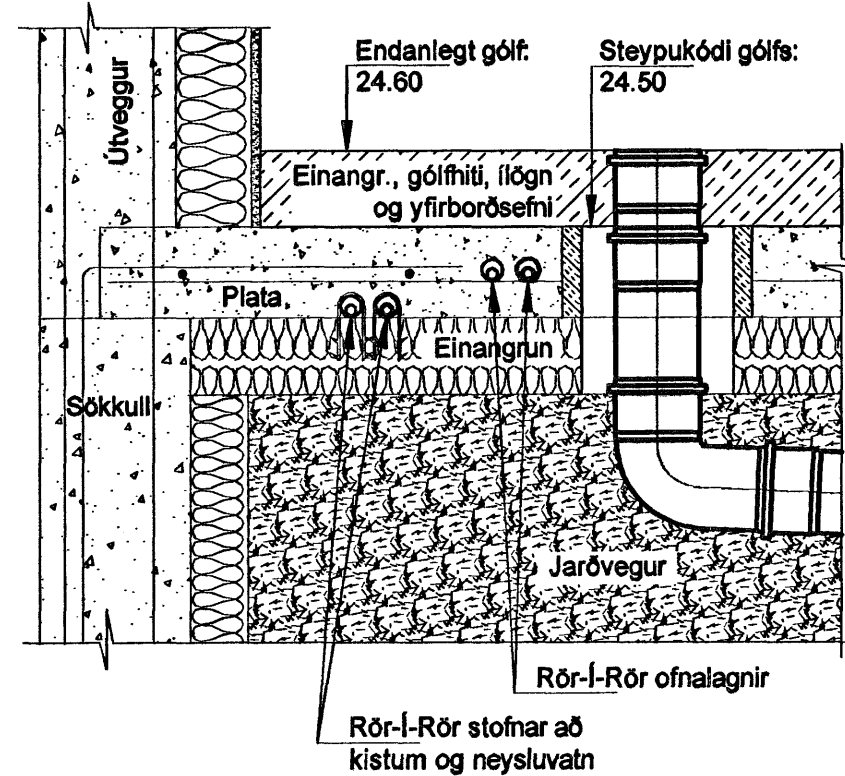
Skematísk sniðmynd yfir frágang helstu lagna undir og í gólfplötu Mkv. 1:10
