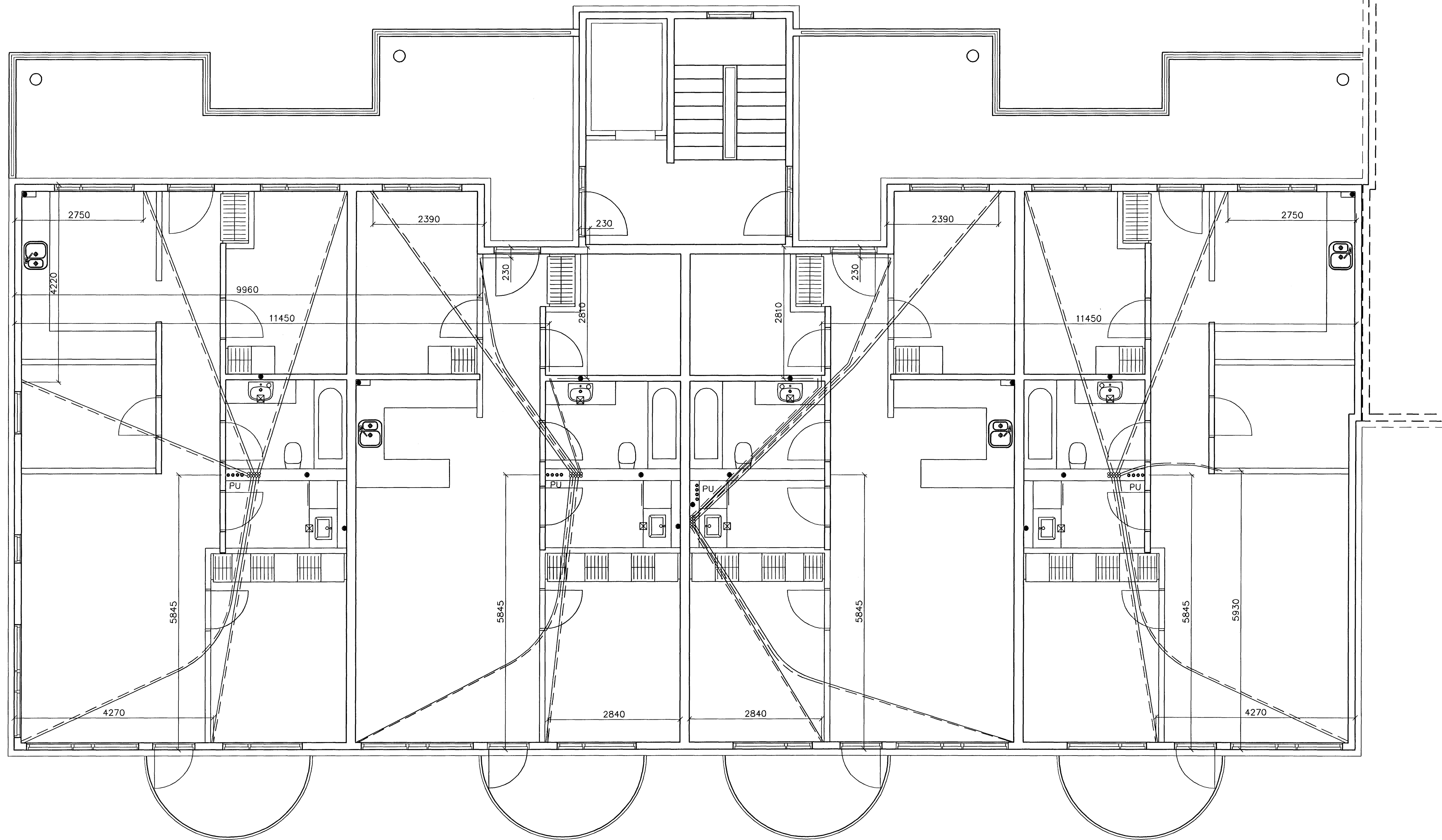
GRUNNMYND 2 HÆÐAR 1:50
