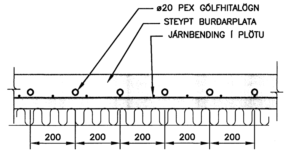
GÓLFHITALAGNIR. SNID MKV. 2 (A1)
