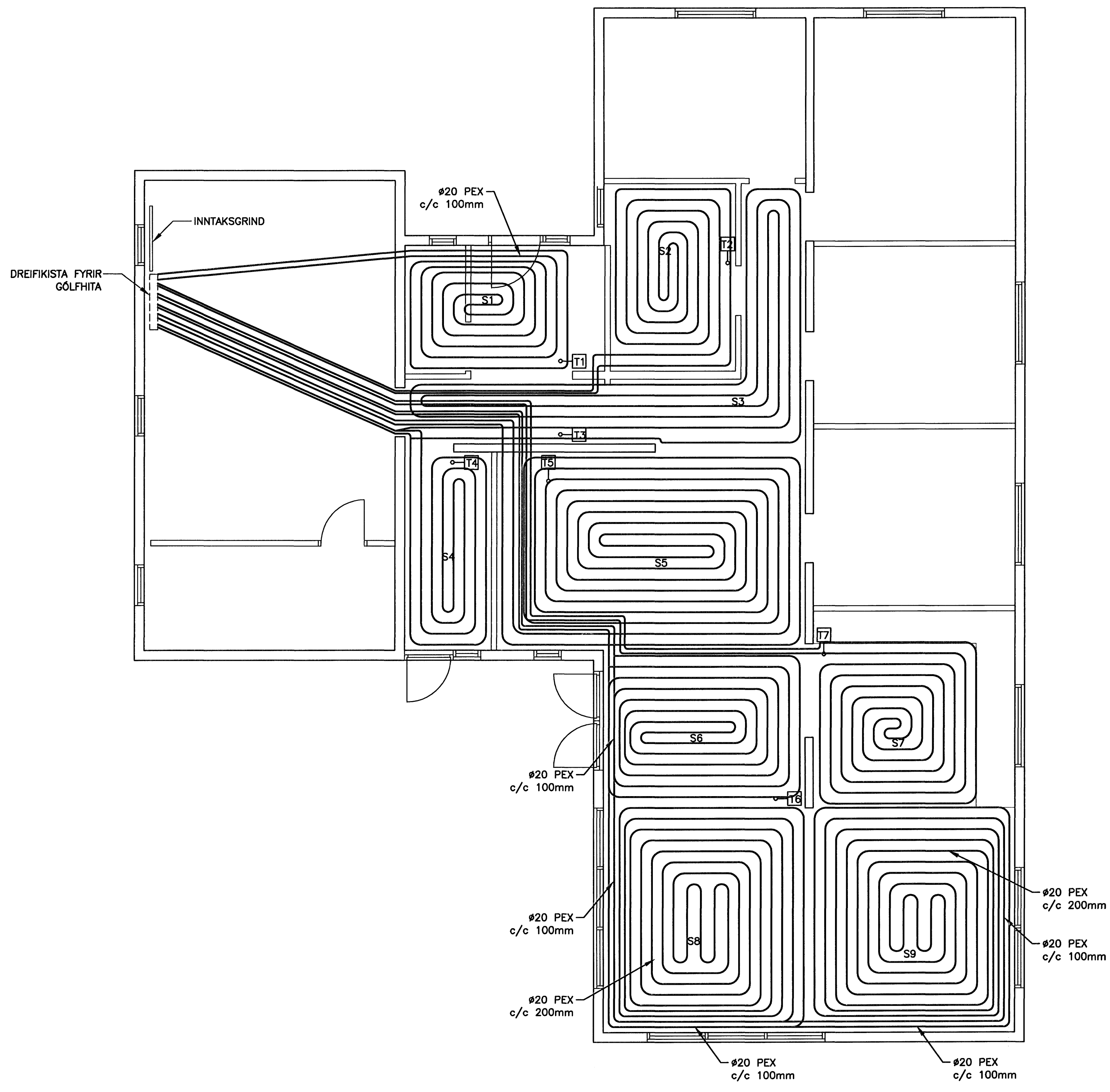
GÓLFHITALAGNIR. GRUNNMYND MKV. 1 (A1)
