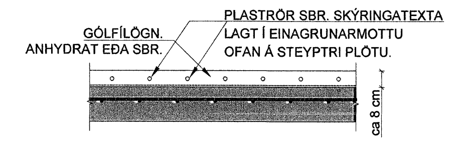
KENNISNIÐ. 1:20 STADSETNING RÖRA Í PLÖTU JARÐHÆÐ
