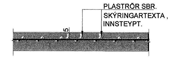
KENNISNIÐ. 1:20 STADSETNING RÖRA Í PLÖTU JARÐHÆÐ
