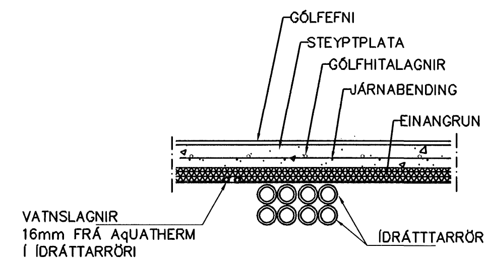
LAGNIR, SNIÐ, 1:20
