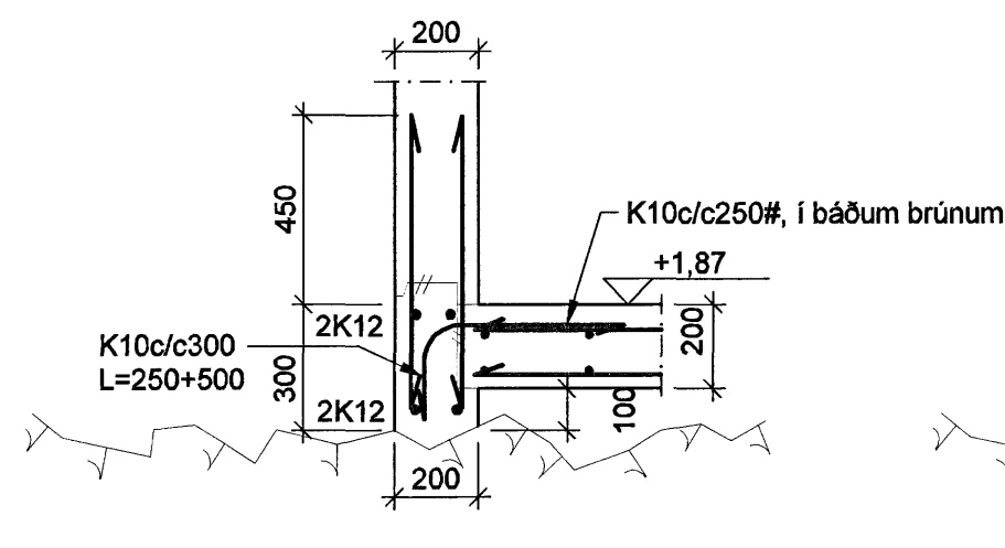
B SNID M. 1: 20
