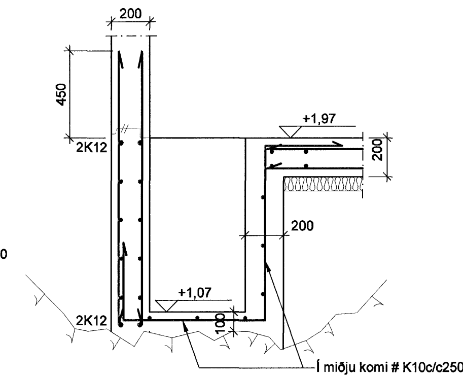
E SNID M. 1: 20
