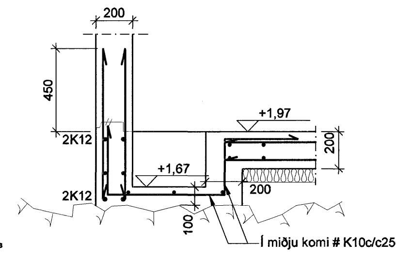
D SNID M. 1: 20
