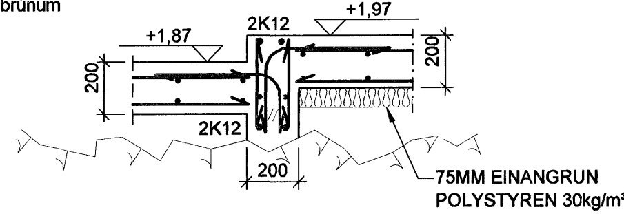
C SNID M. 1: 20
