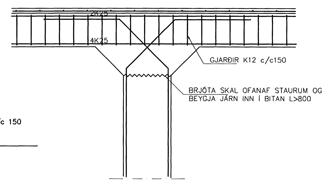
ASYND A-A Á STAURA 1:20
