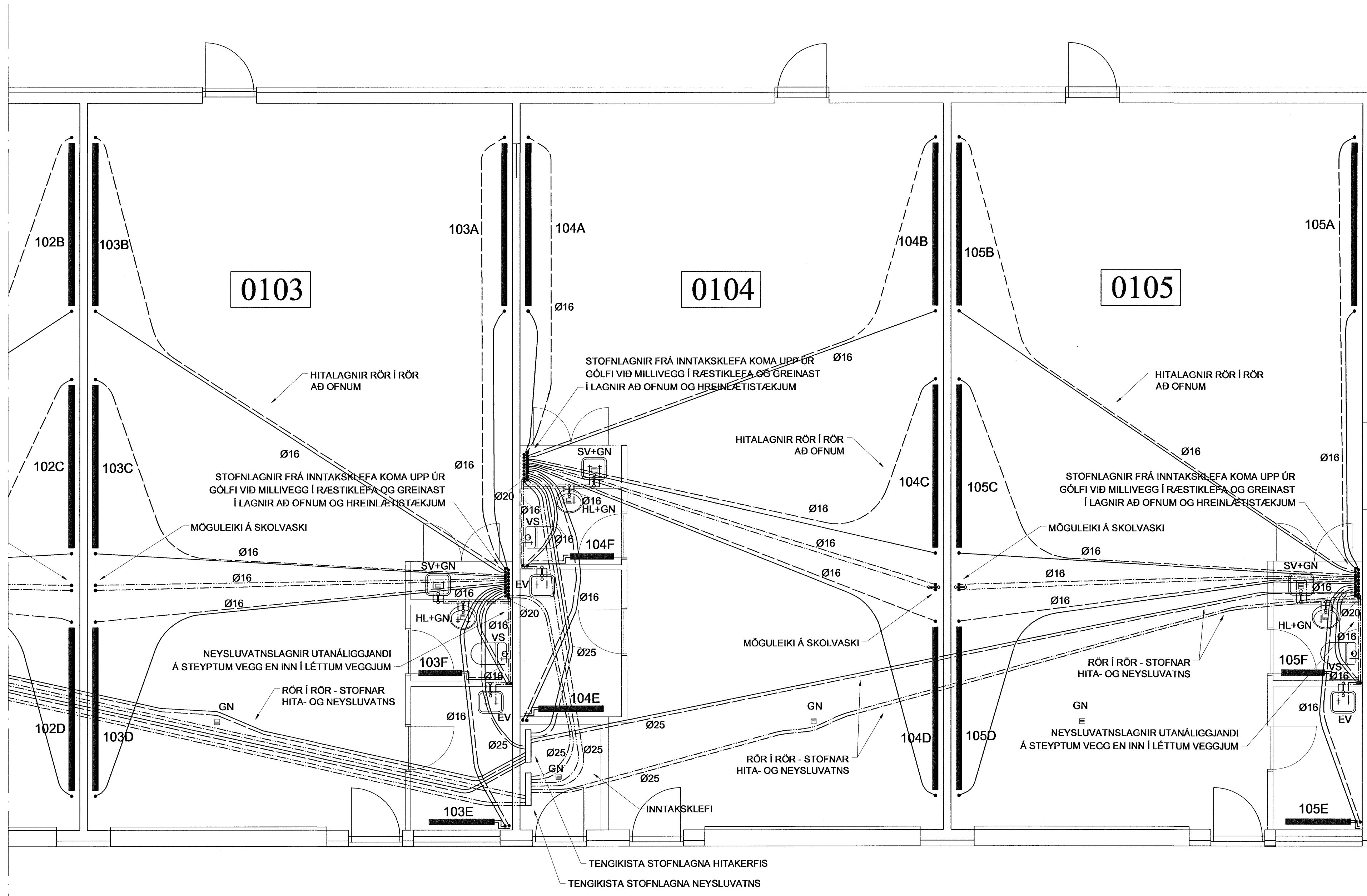
GRUNNMYND SUÐURHLUTA HÚSS 1:50
