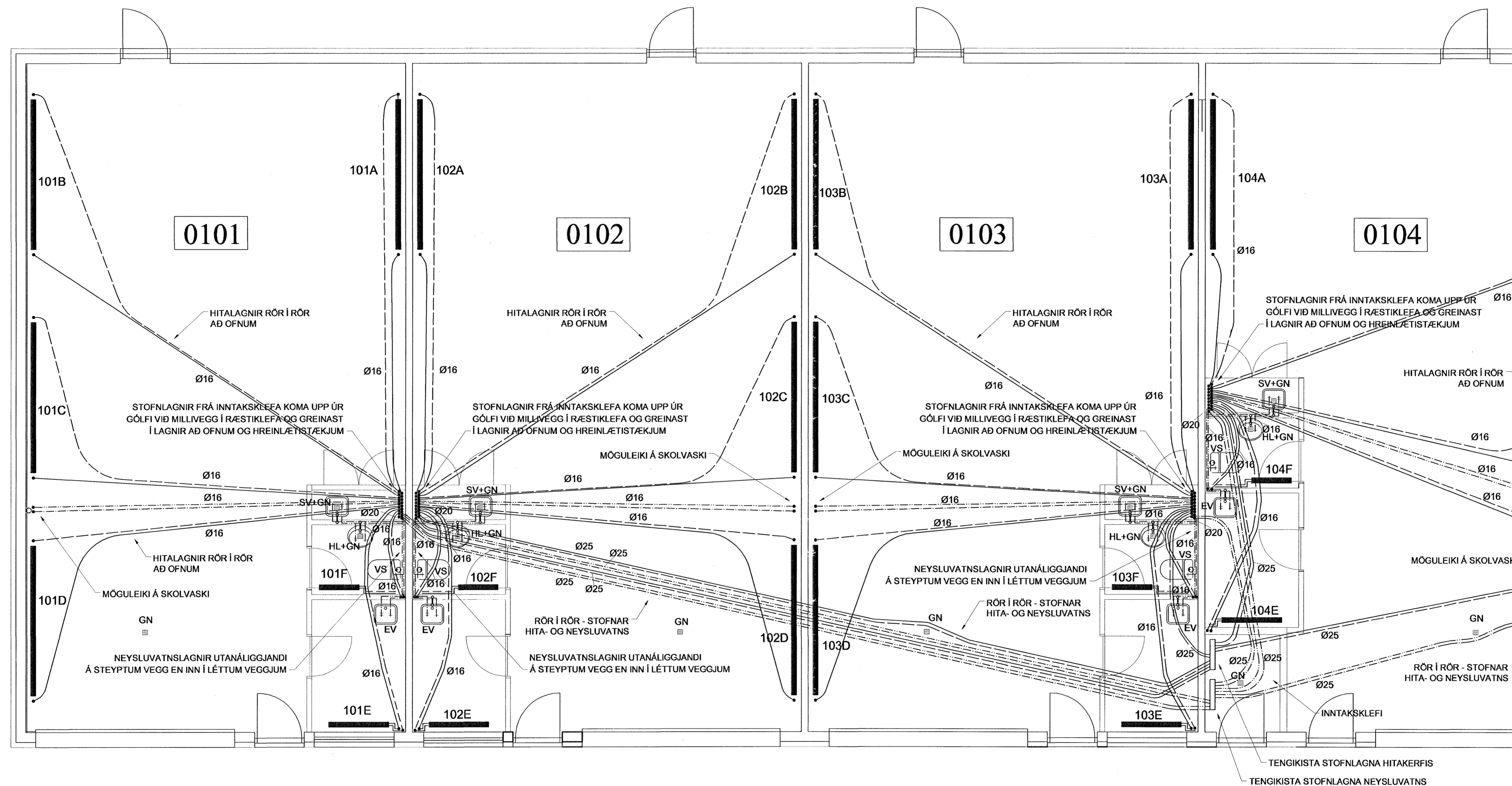
GRUNNMYND NORÐURHLUTA HÚSS 1:50
