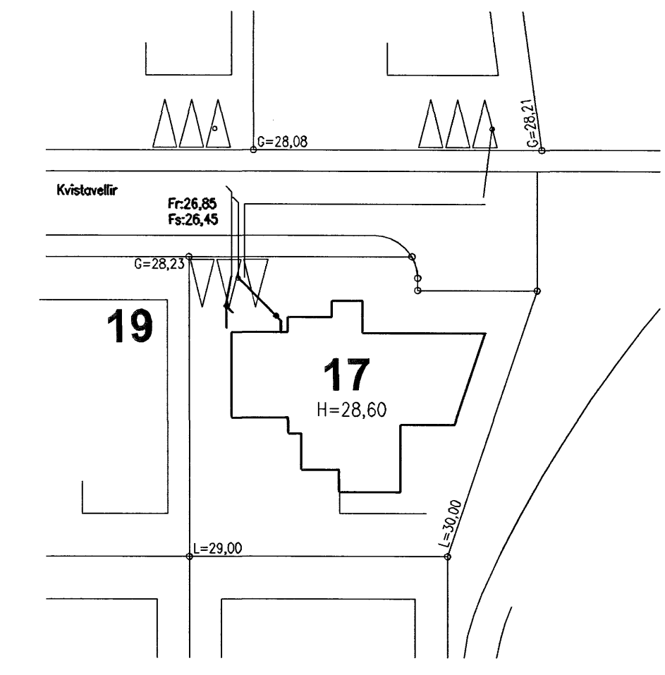
Afstöðumynd 1:500
