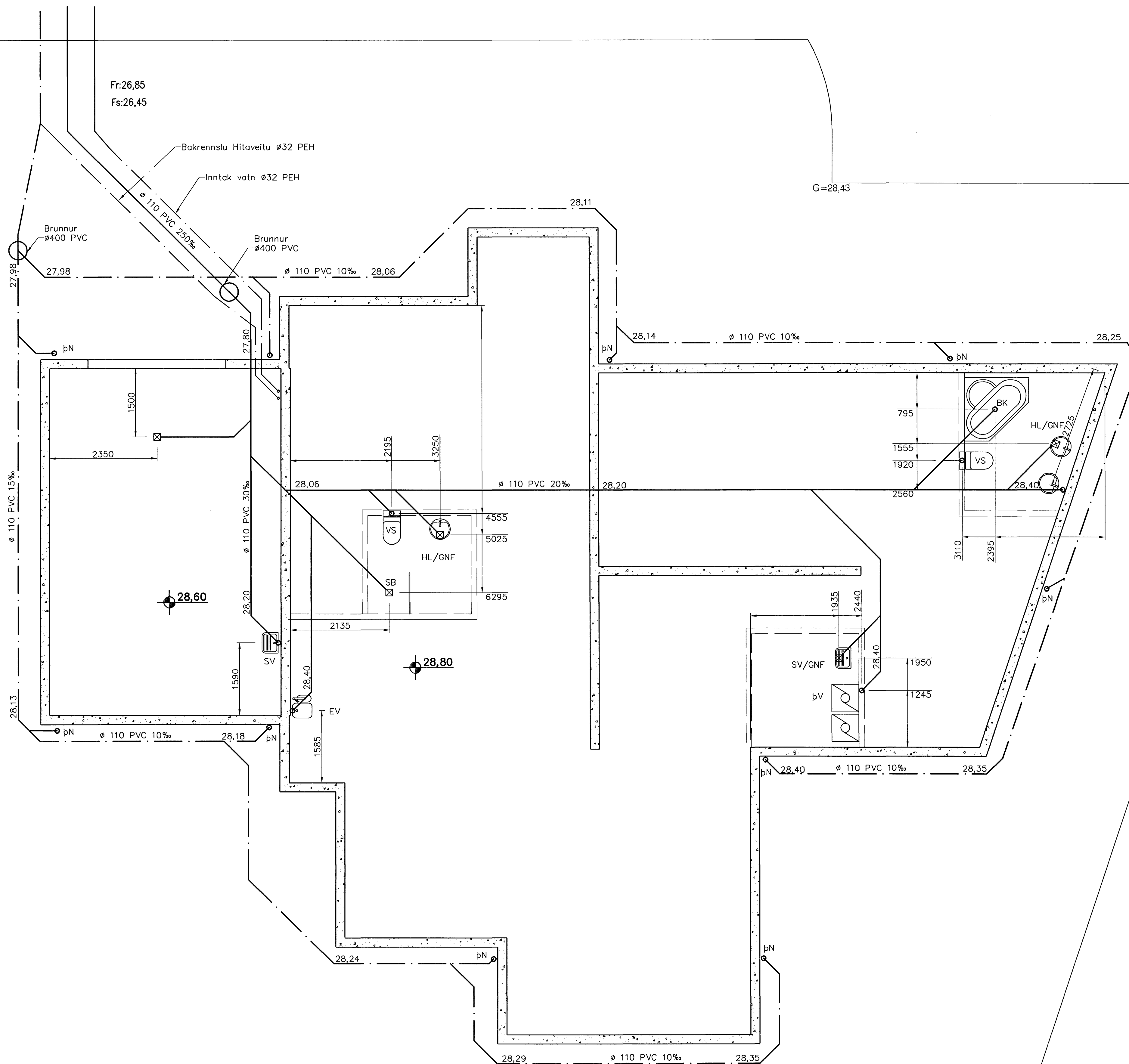
Grunnlagnir 1:50
