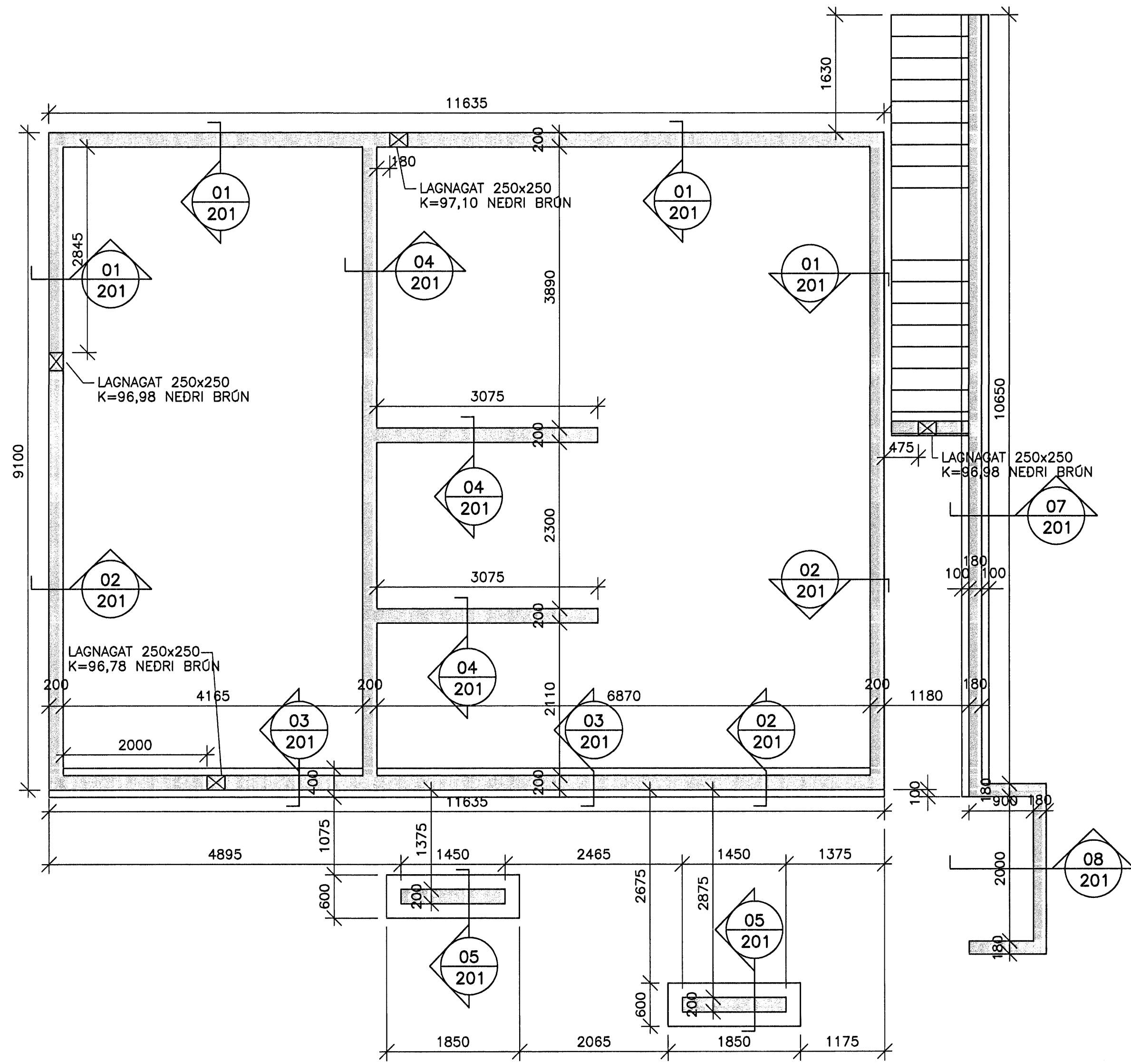
SÖKKULL GRUNNMYND. 1:50
