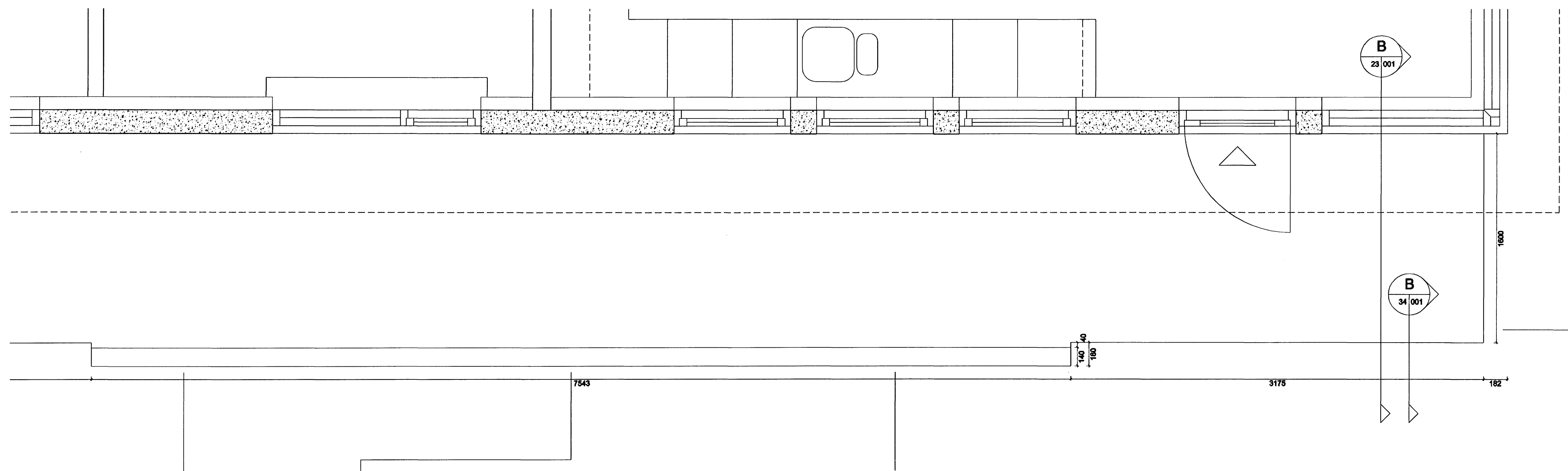
Grunnmynd svala, 2. hæð 1: 20
