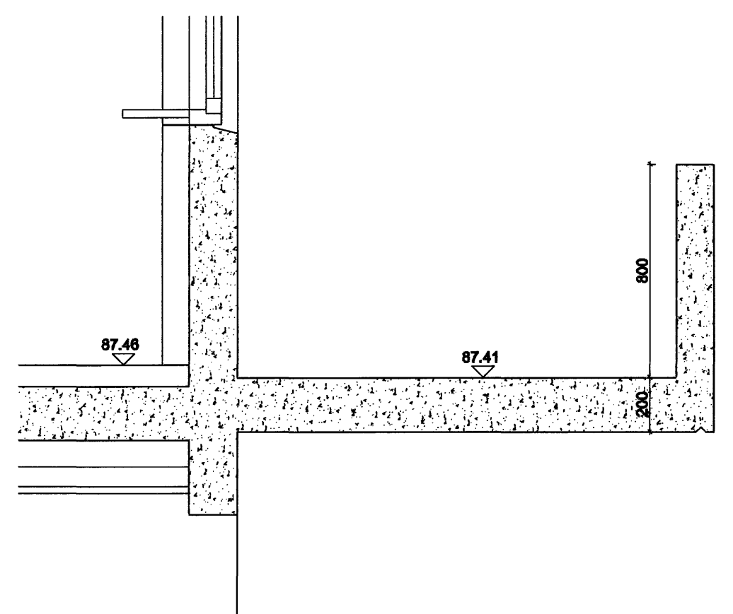
A 23/001 Skurður A 1: 20
