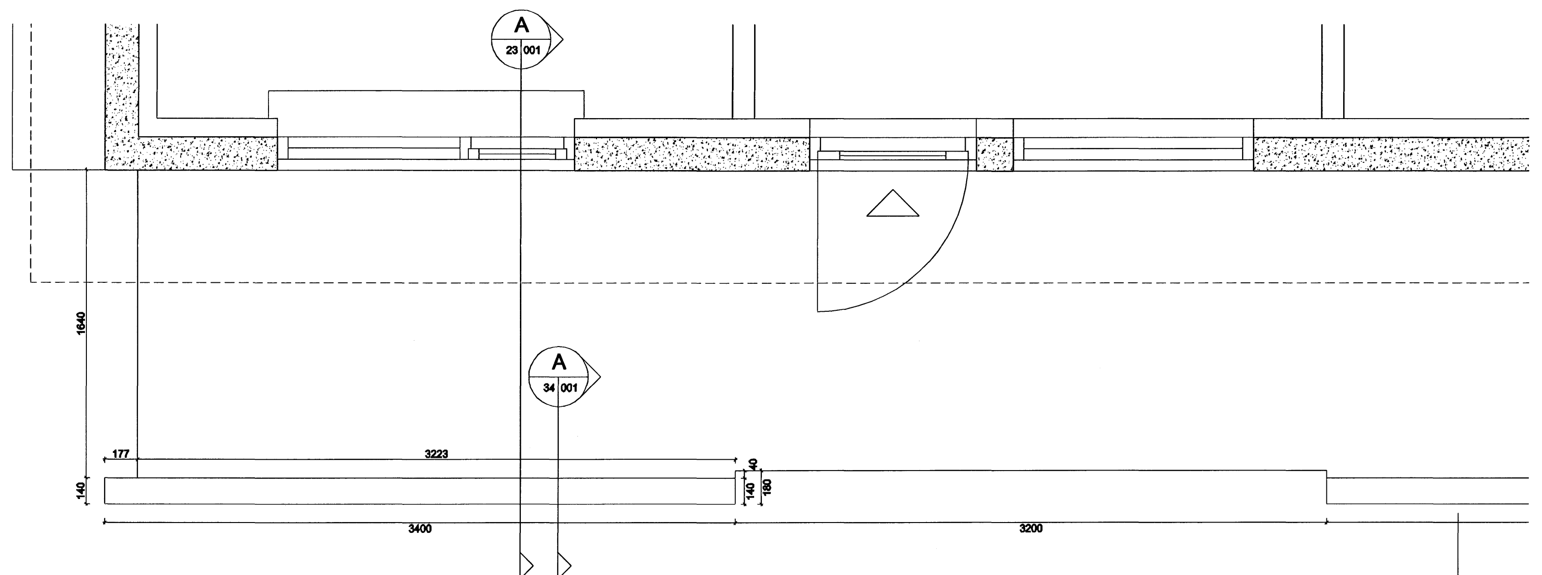
Grunnmynd svala, 2. hæð 1: 20
