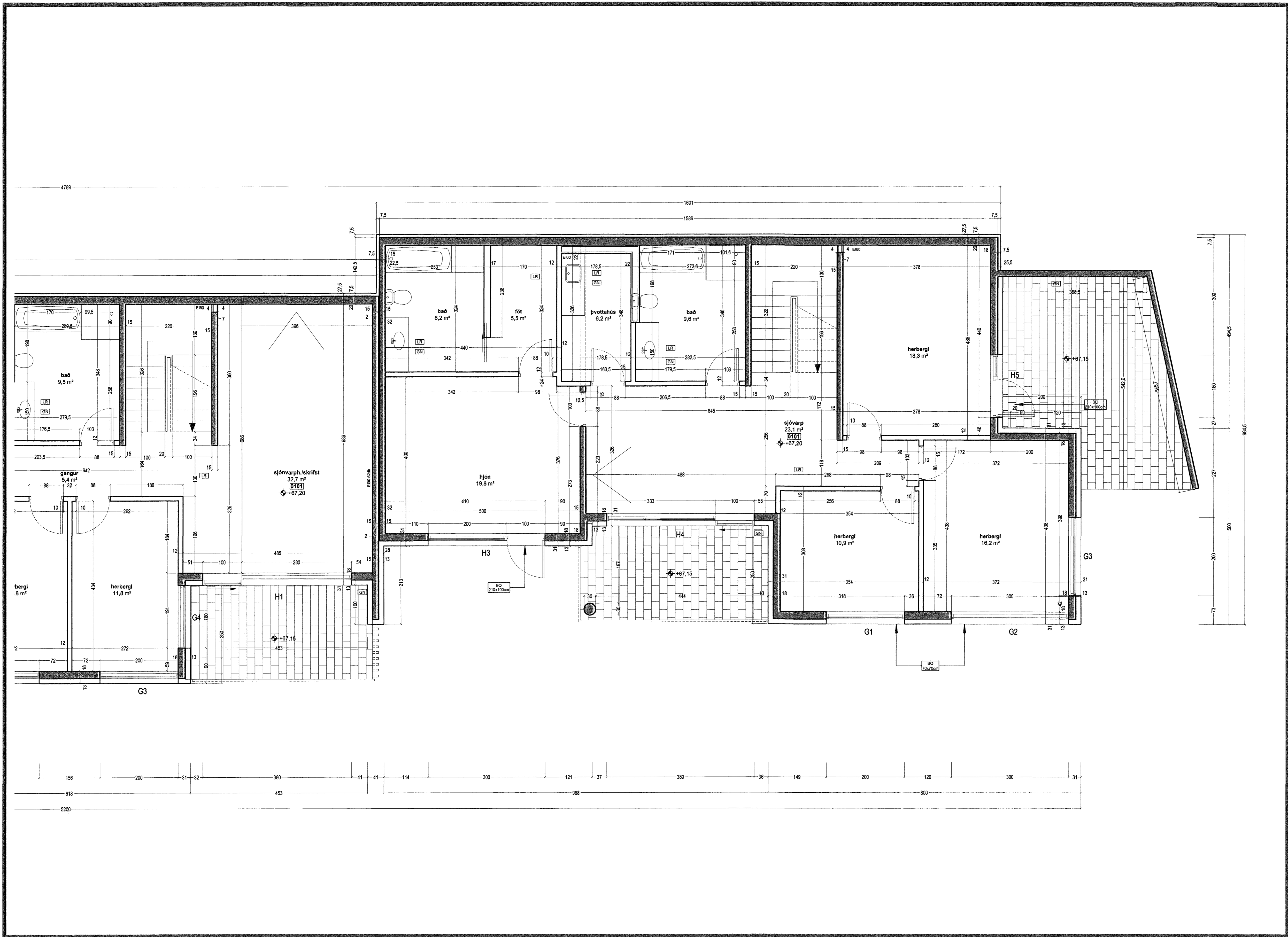
Grunnmynd 1.hæð 1:50
