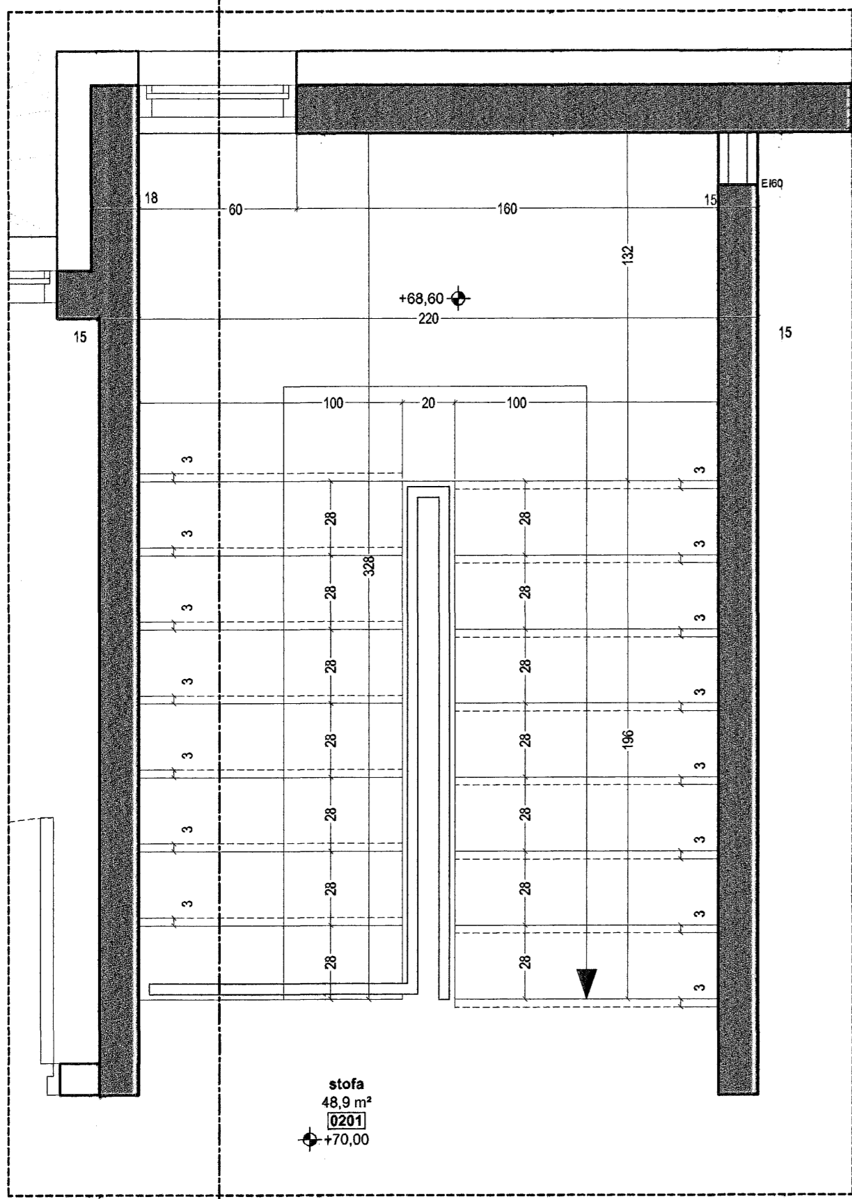
Stigateikning Grunnmynd 2.hæð 1:20
