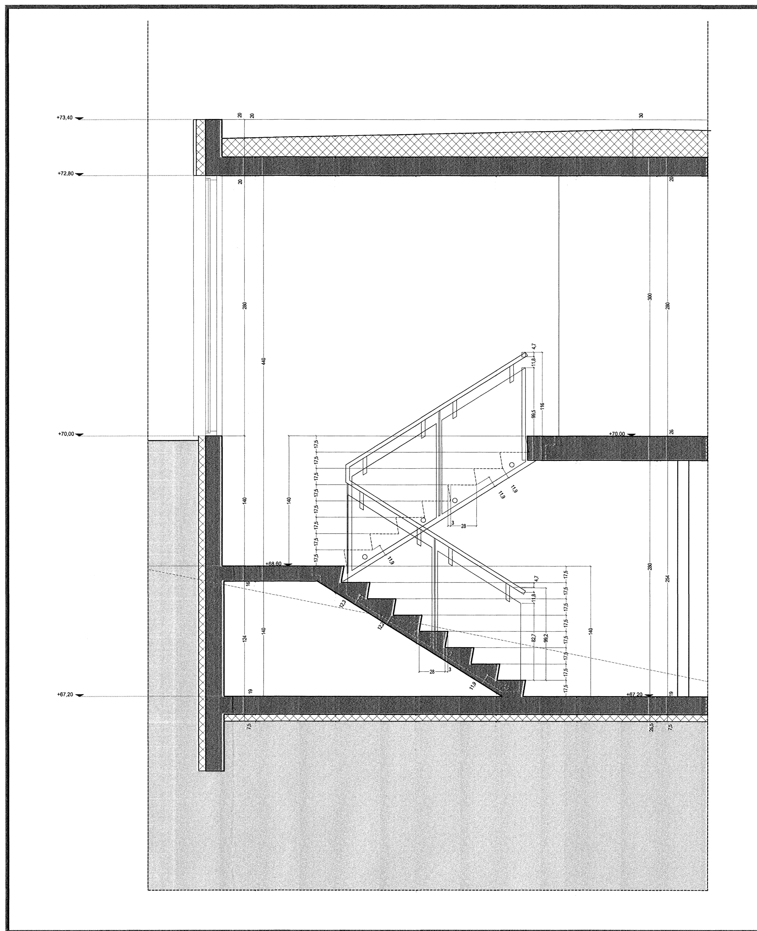
Stigateikning Snið S2 1:20
