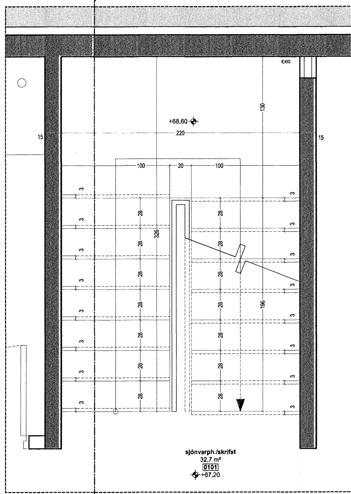
Stigateikning Grunnmynd 1.hæð 1:20
