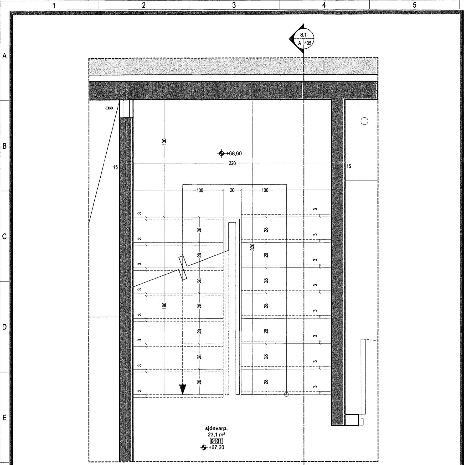
Stigateikning Grunnmynd 1.hæð 1:20
