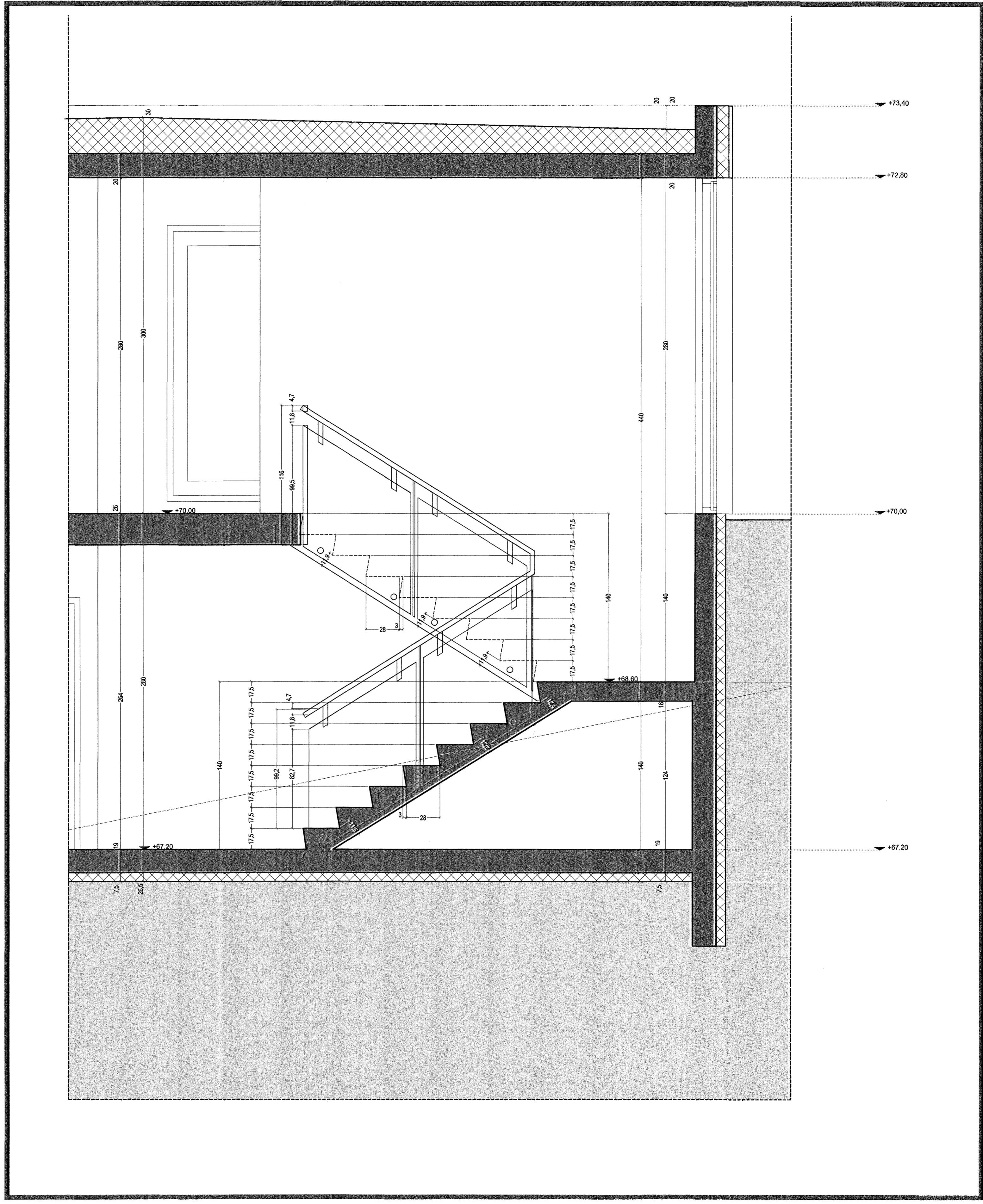
Stigateikning Snið S1 1:20
