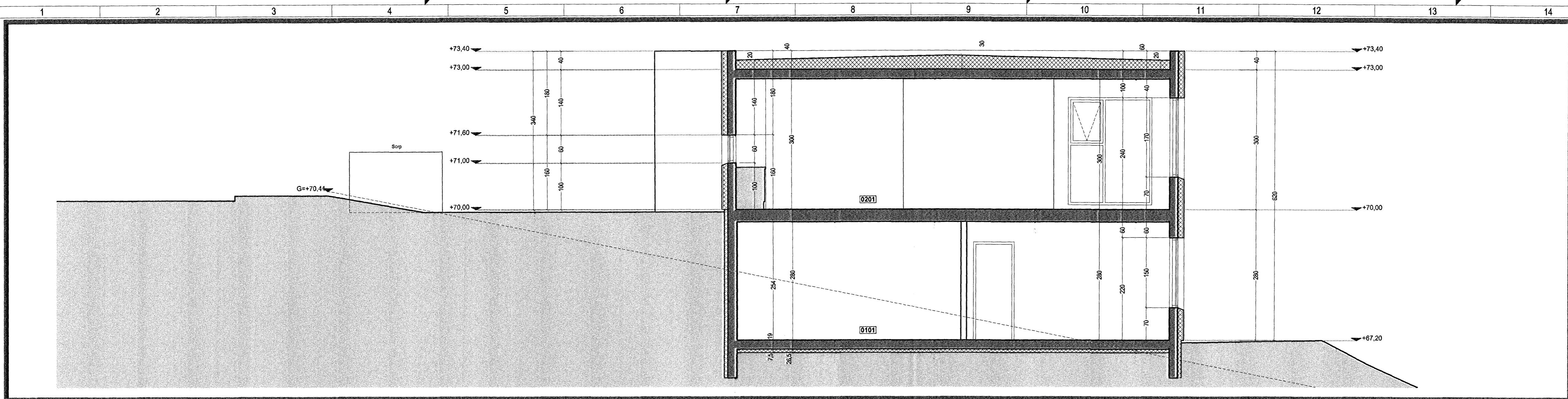
Snið S1 1:50
