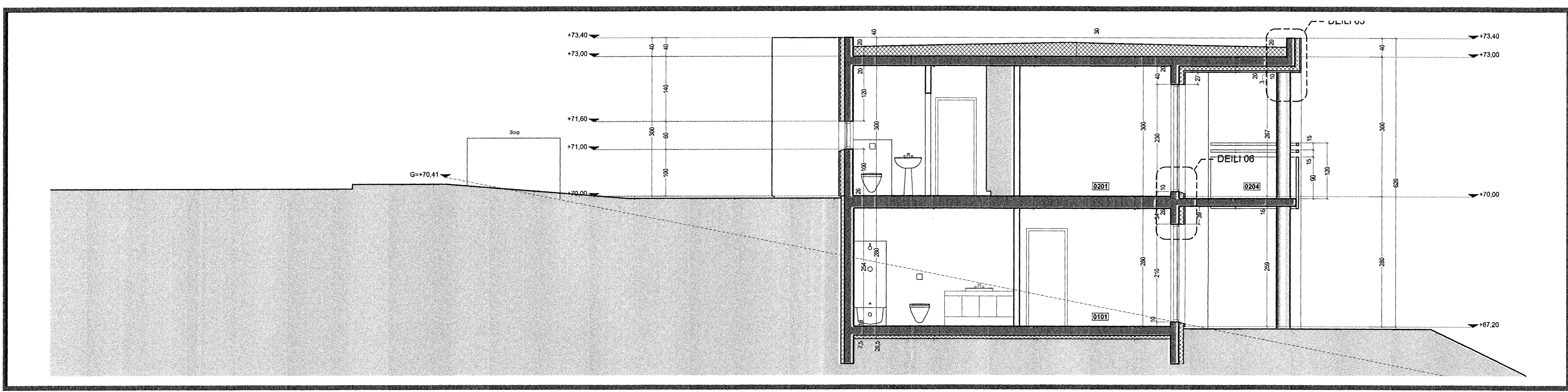
Snið S3 1:50
