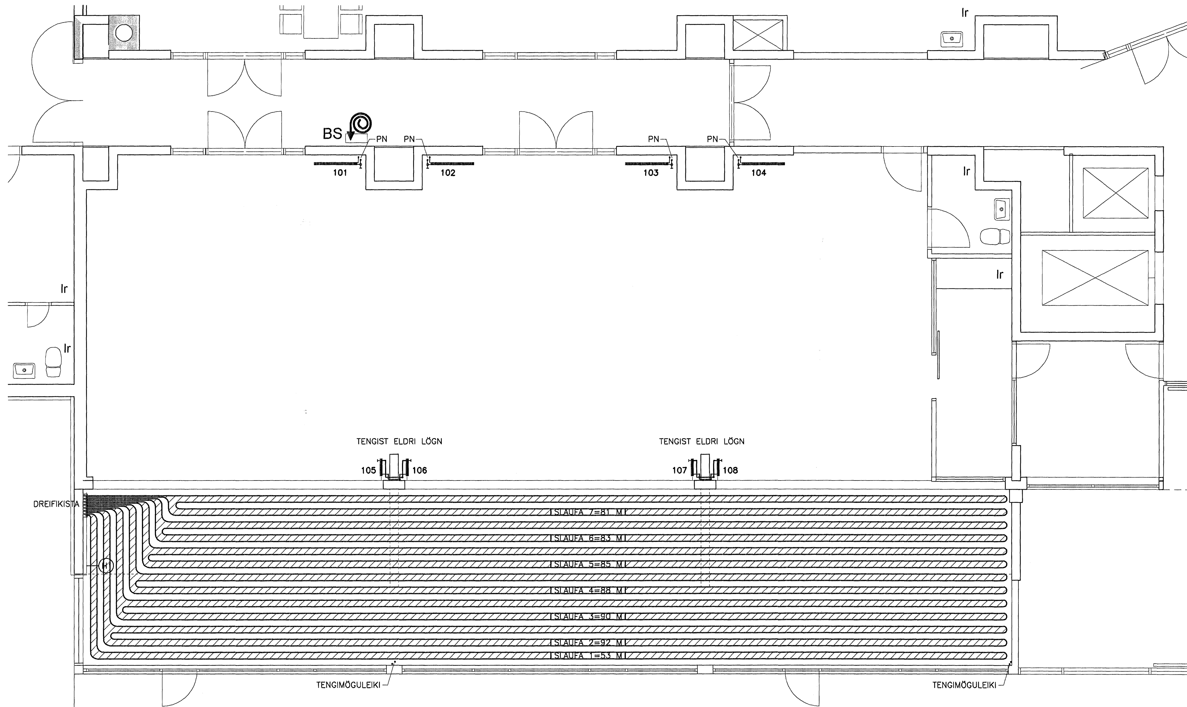
GRUNNMYND, 1:50
