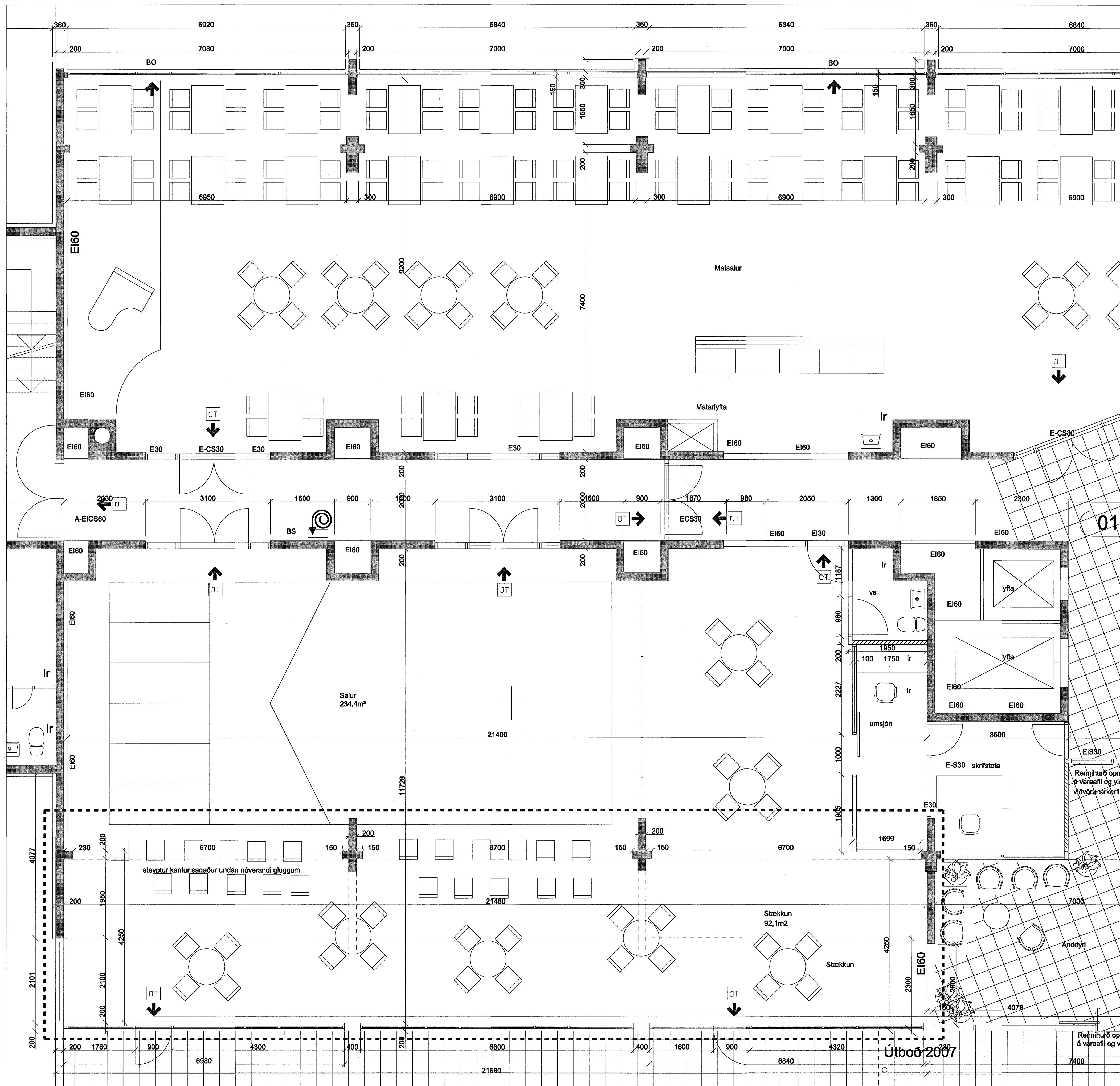
GRUNNMYND 1:HÆÐAR 1:50
