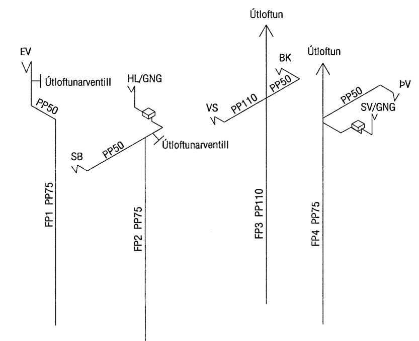
Fallpípur 1:50
