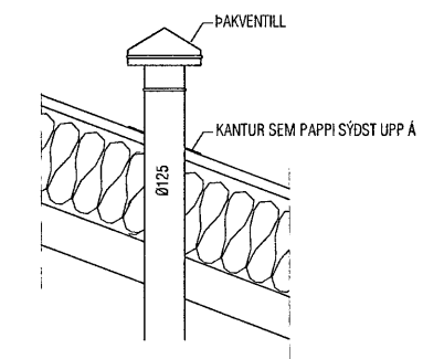
DÆMIGERÐ LOFTRÆSING RÝMA. M1:20
