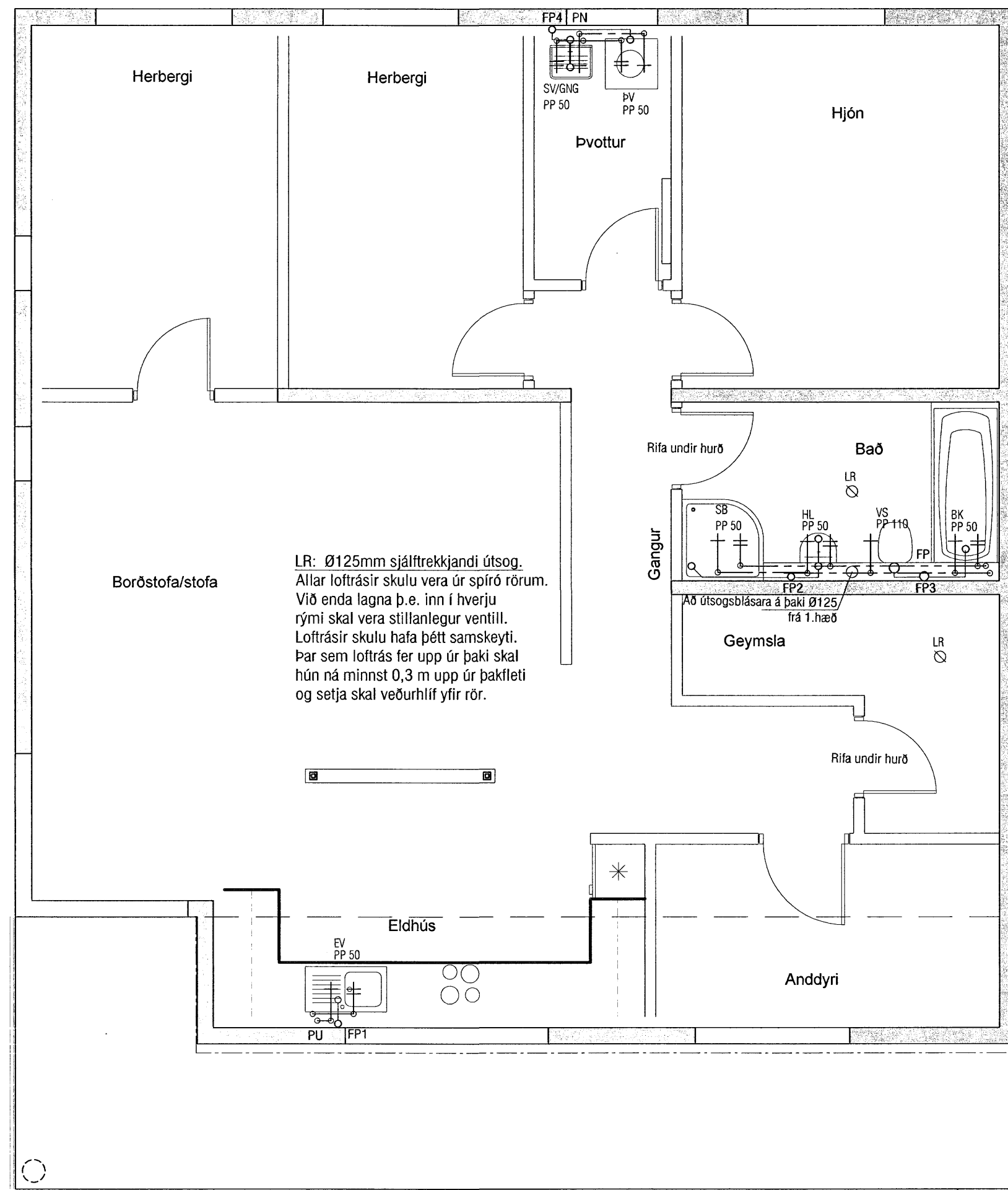
Grunnmynd 2.hæð 1:50
