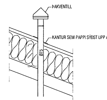
DÆMIGERÐ ÚTLOFTUN RÝMA. M1:20
