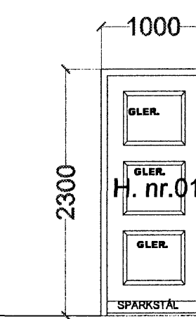
ÚTIDYRAHURÐIR 10 STK HURÐ OPNIST INN V. 15 STK HURÐ OPNIST INN H.
