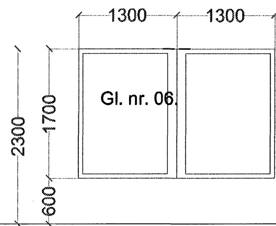
10 STK. HORNGLUUGGAR STOFA..
