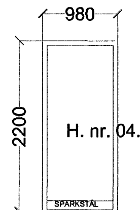
1. STK. BRUNASTÚKA. ELDV.HURÐ. EI-CS-30. OPNIST ÚT H.
