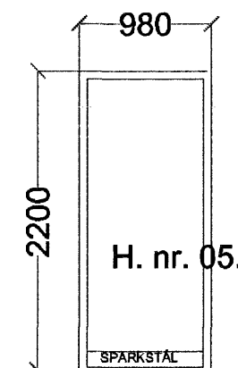
1. STK. BRUNASTÚKA. ELDV.HURÐ. EI-CS-60. OPNIST INN H.
