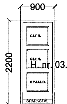
Bílakjallari. 1. STK HURÐ OPNAST VINSTRI ÚT.. STJÓRNK. VATSK. 1 STK opnist inn HÆGRI.
