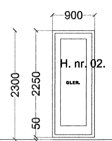
10 STK. SVALAH. OP. ÚT H. 10 STK. SVALAH. OP. ÚT V.
