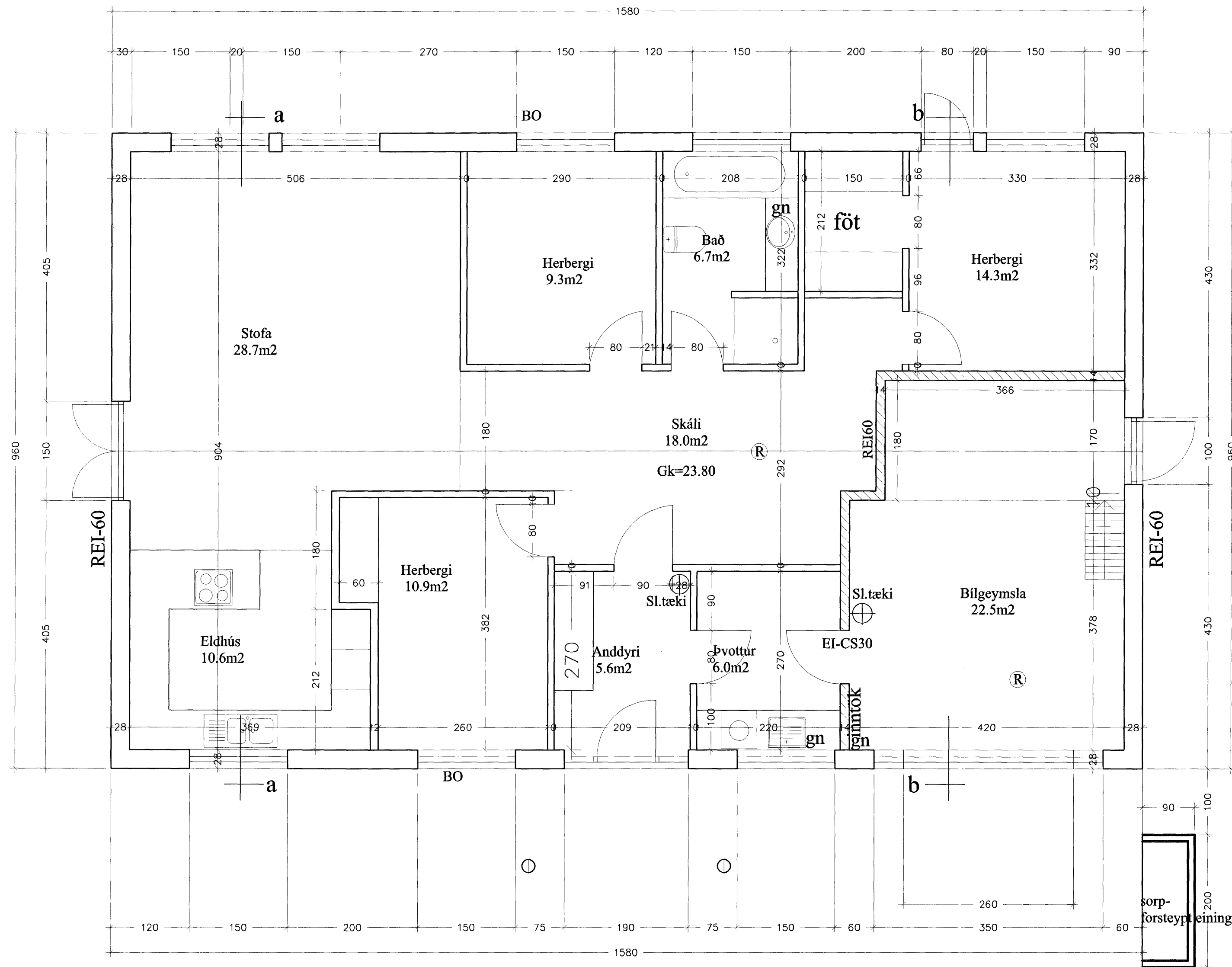
GRUNNMYND 1.HÆÐ 1:50
