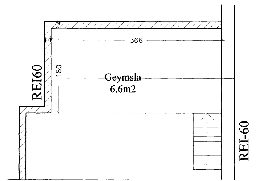
GRUNNMYND MILLIÖSTANNA 1:50
