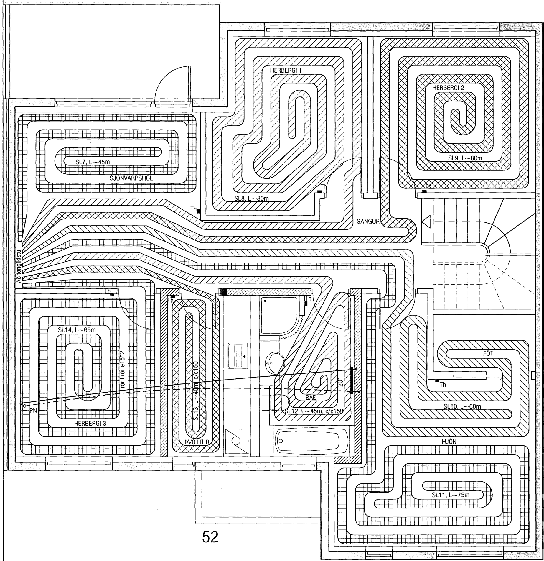
Grunnmynd 2.hæð 1:50
