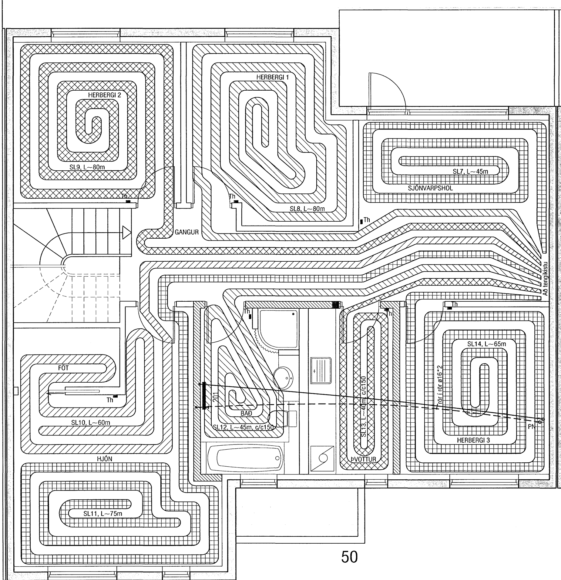
Grunnmynd 2.hæð 1:50
