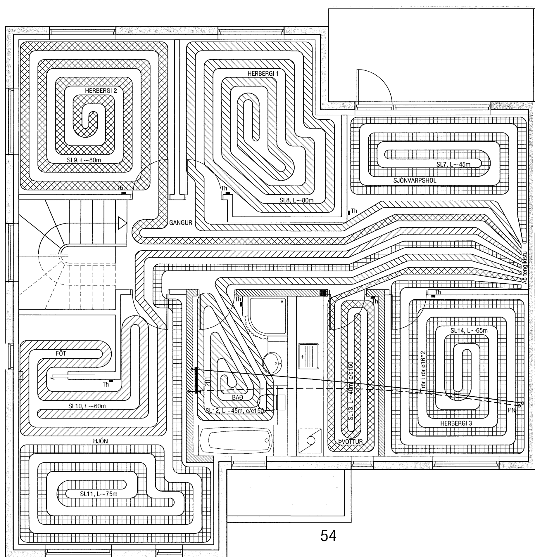
Grunnmynd 2.hæð 1:50
