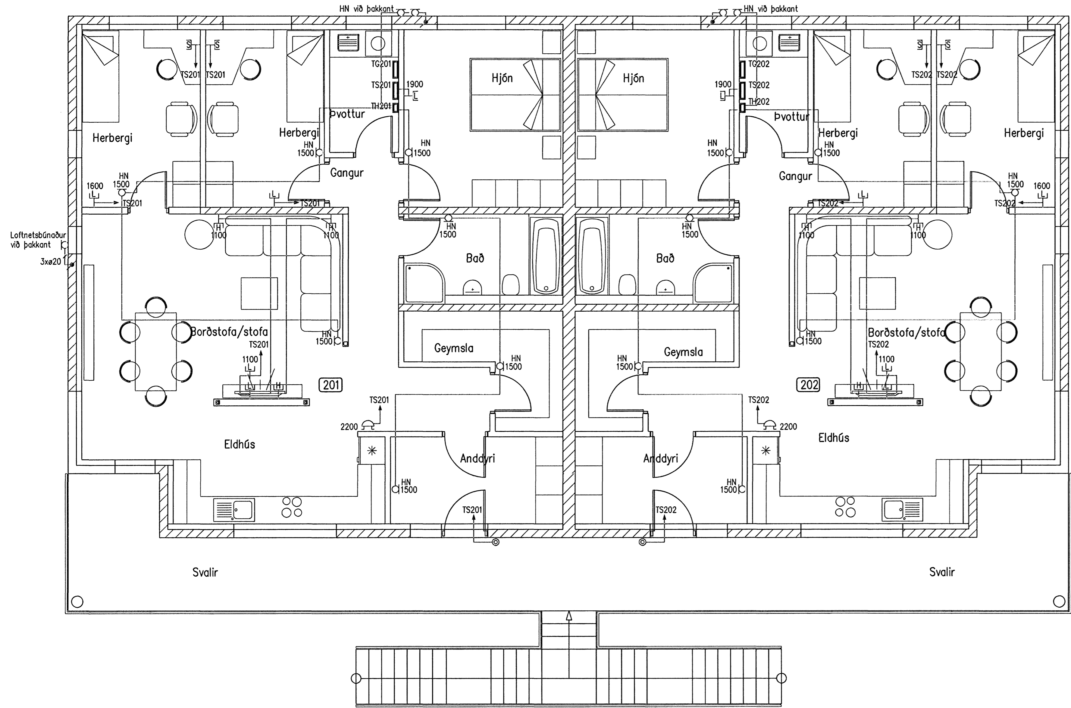
Grunnmynd 2. hæð, 1:50
