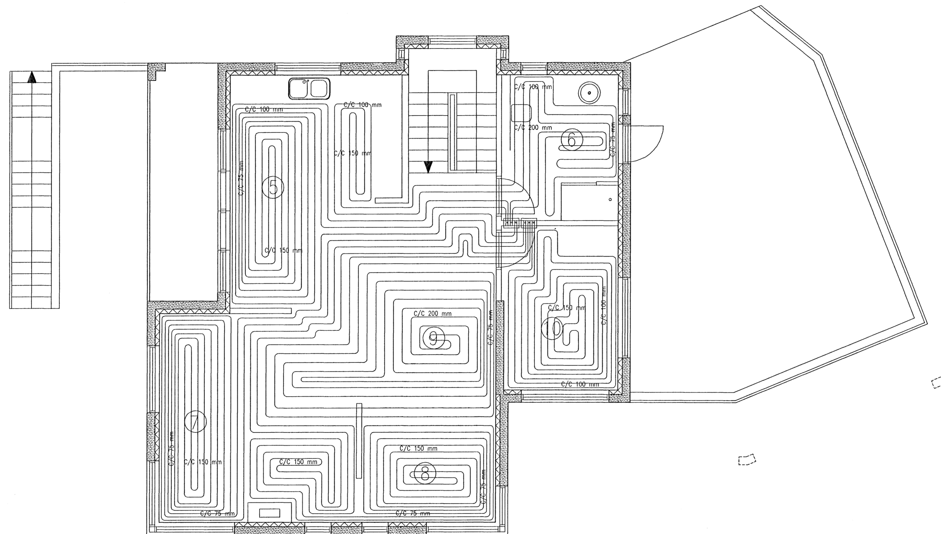
GRUNNMYND GÓLFHITALAGNA 2.HÆÐAR 1:50
