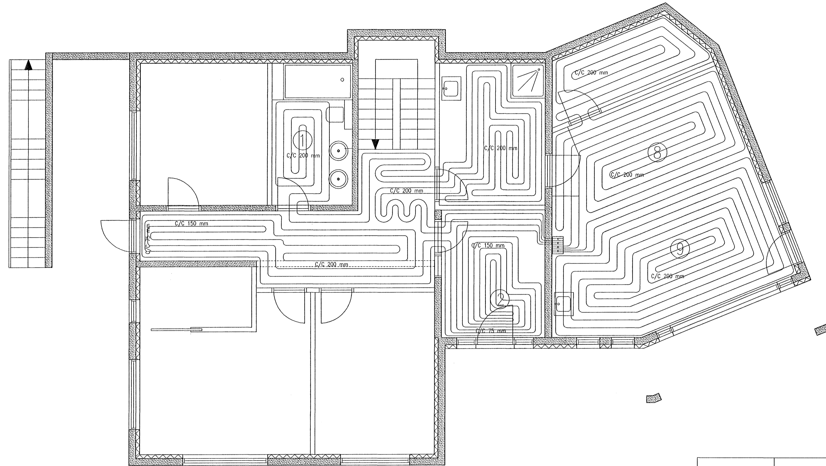
GRUNNMYND GÓLFHITALAGNA 1.HÆÐAR 1:50
