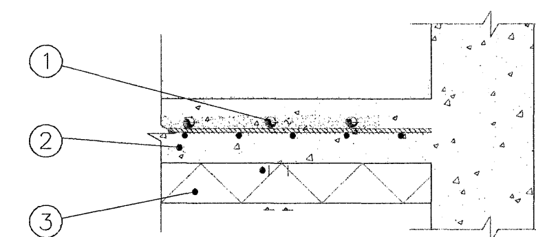
SNID Í BOTNPLÖTU MKV. 1:10
