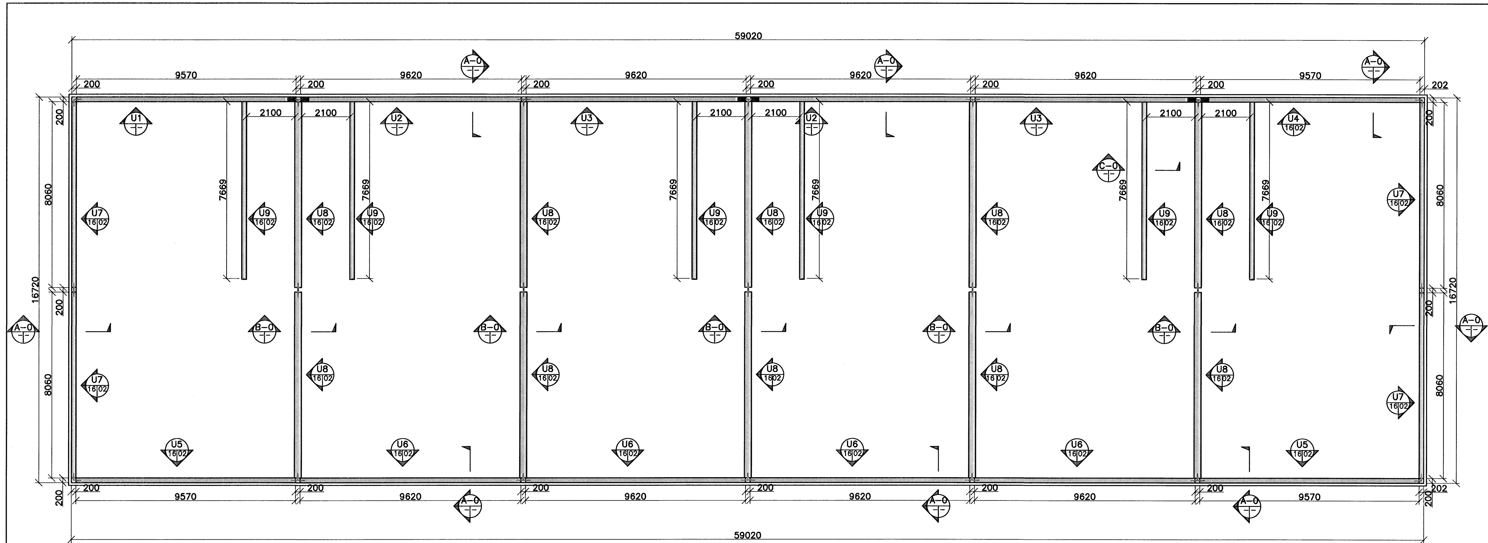
Grunnmynd sökkuls 1:100
