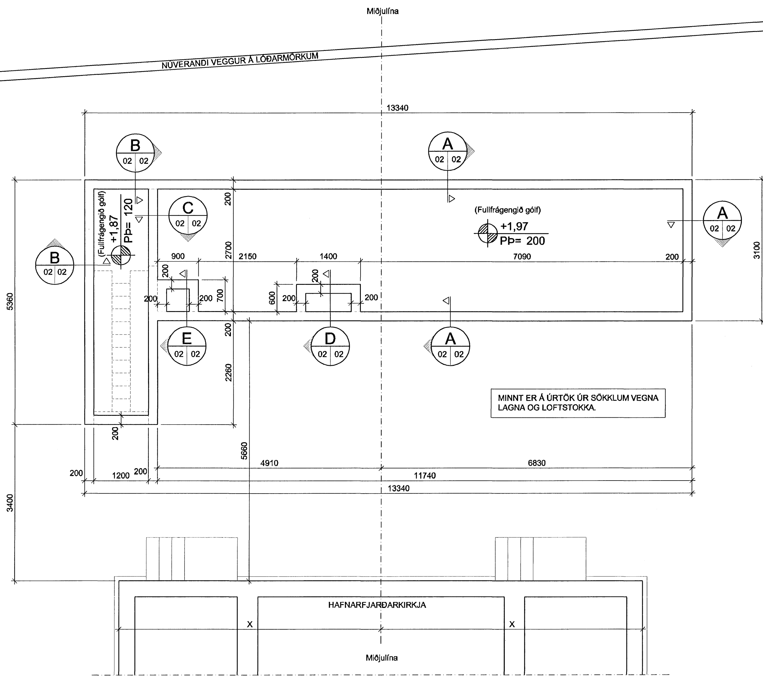
GRUNNMYND UNDIRSTAÐA MKV: 1:50
