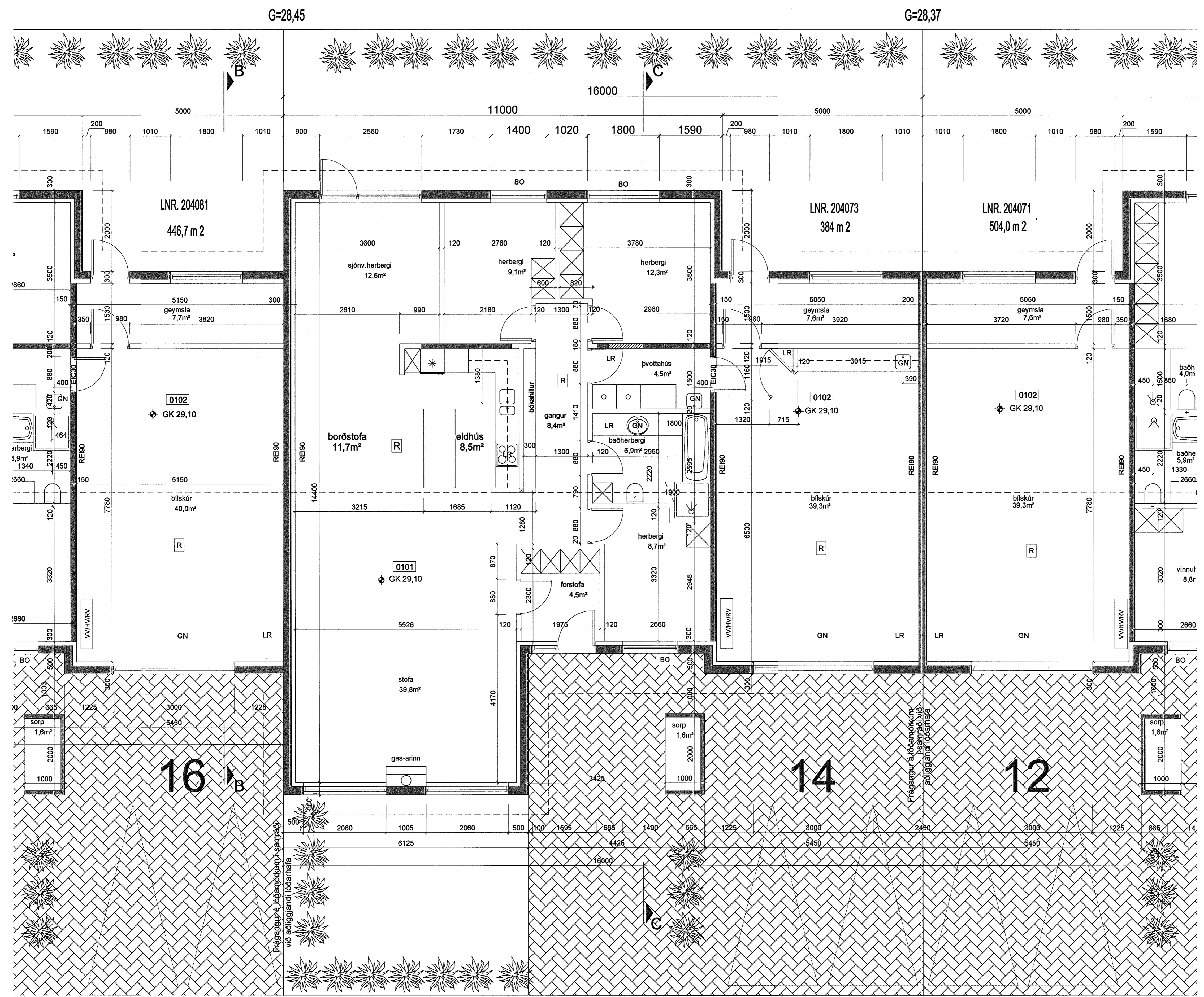
GRUNNMYND 1:50
