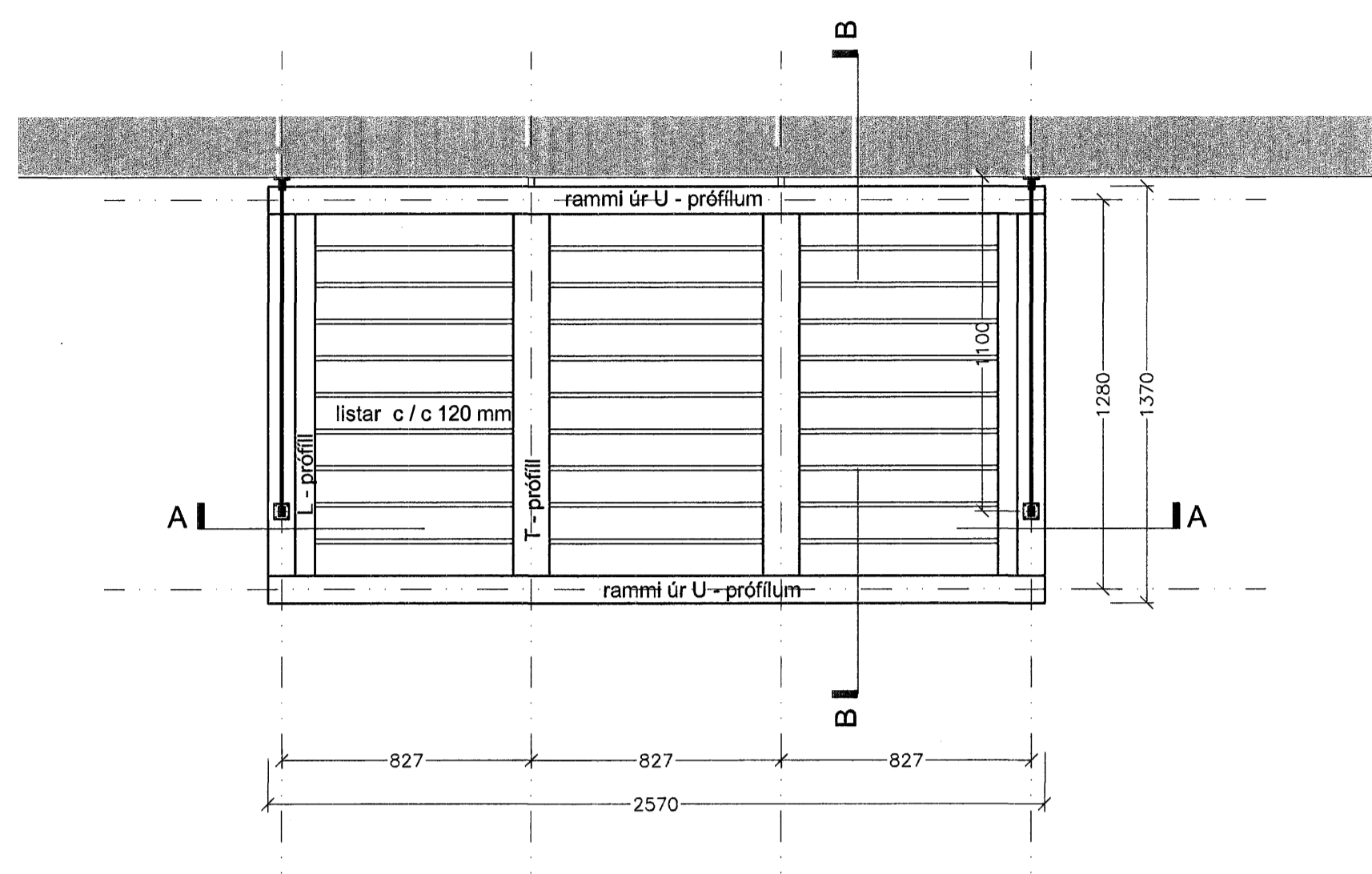
SKYGGNI M 1:20 GRUNNMYND
