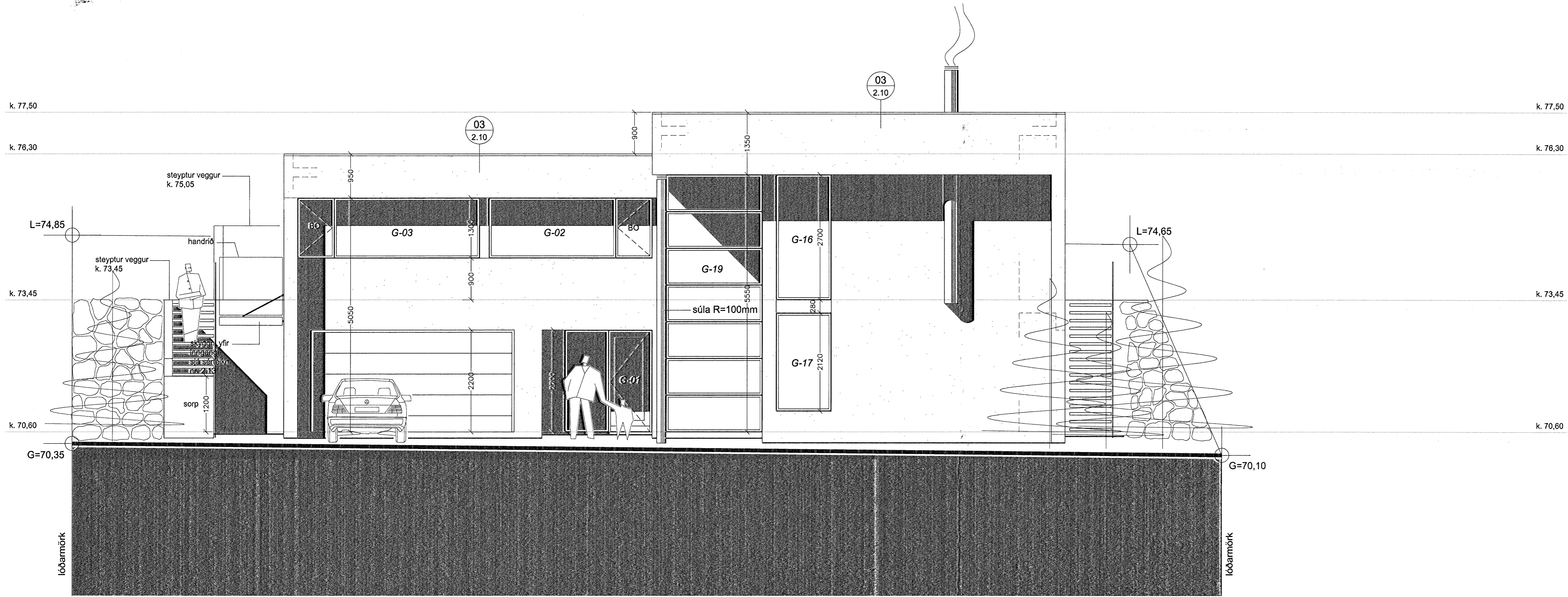
ÚTLIT NORÐAUSTUR M 1:50
