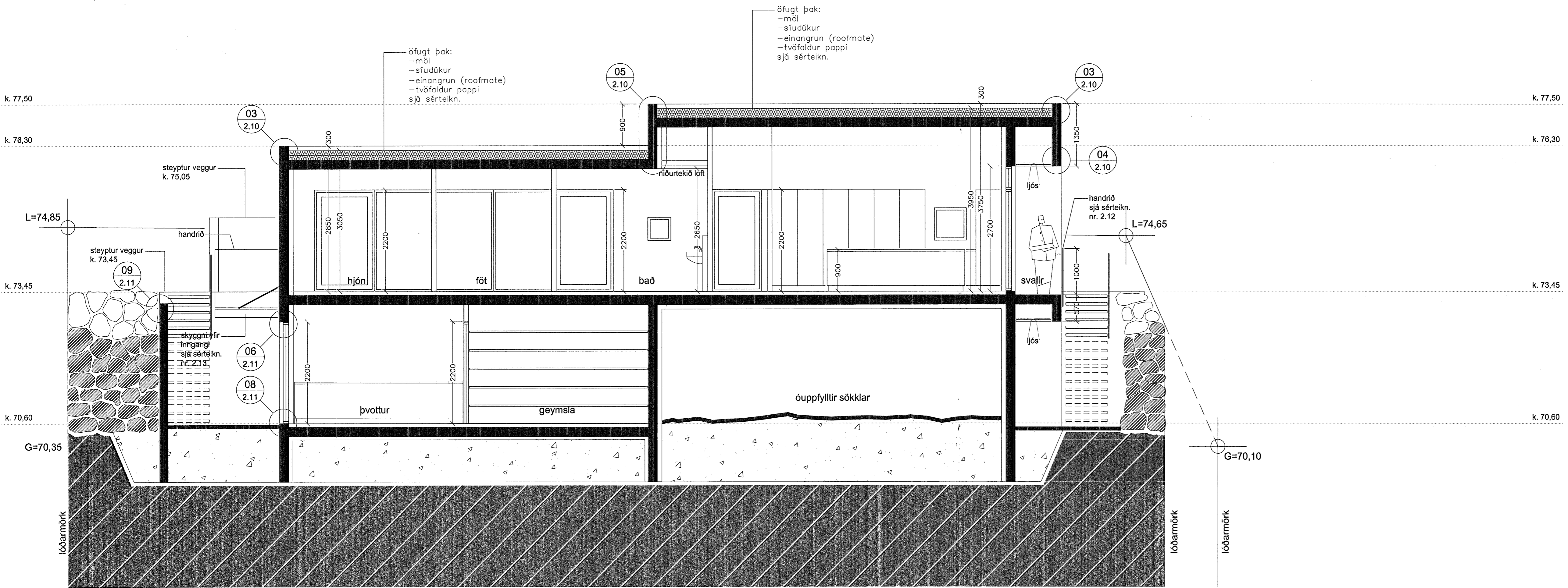
SNEIÐING C - C M 1 : 50
