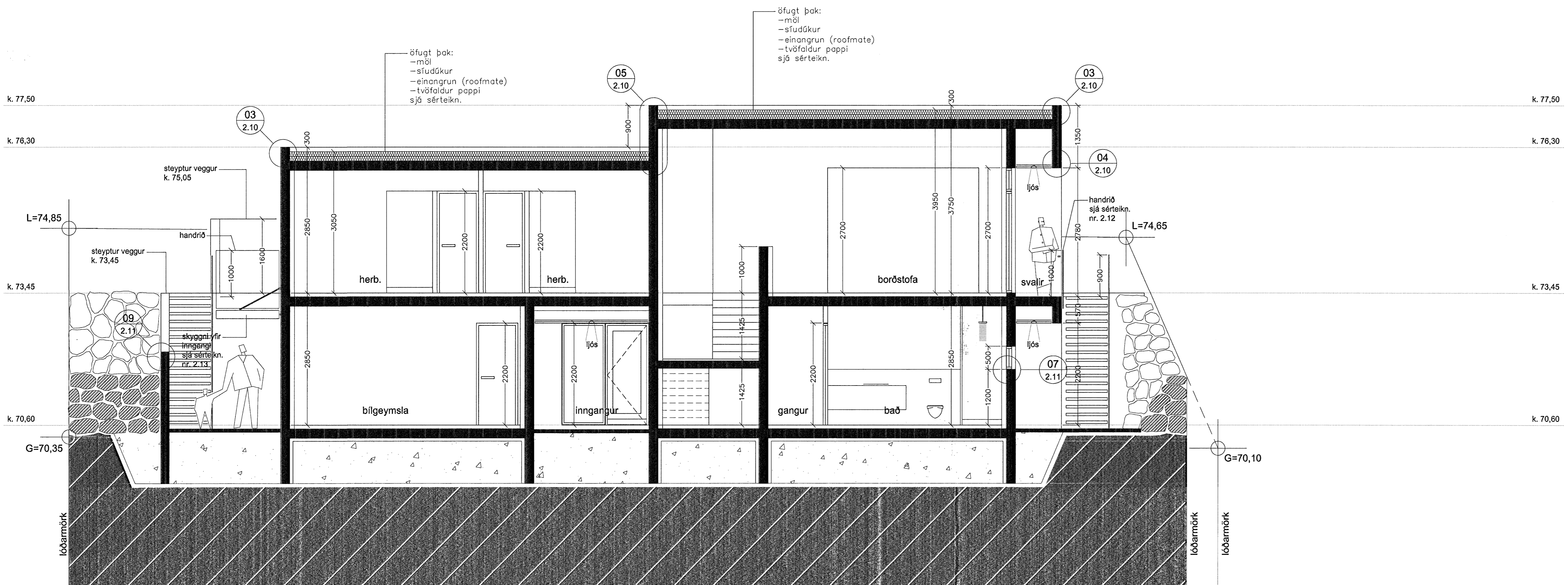
SNEIÐING A - A M 1:50
