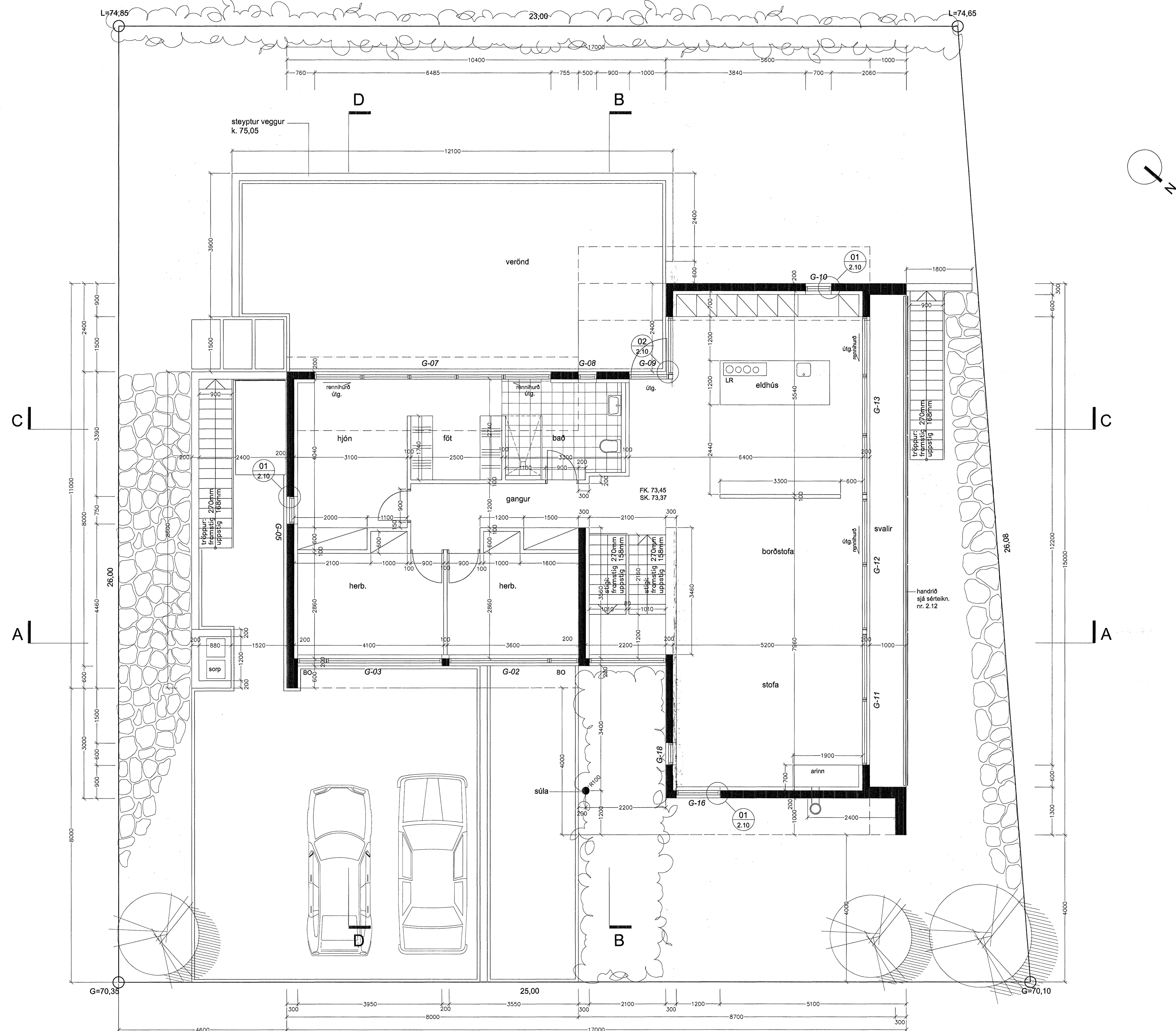
GRUNNMYND EFRI HÆÐ M 1 : 50
