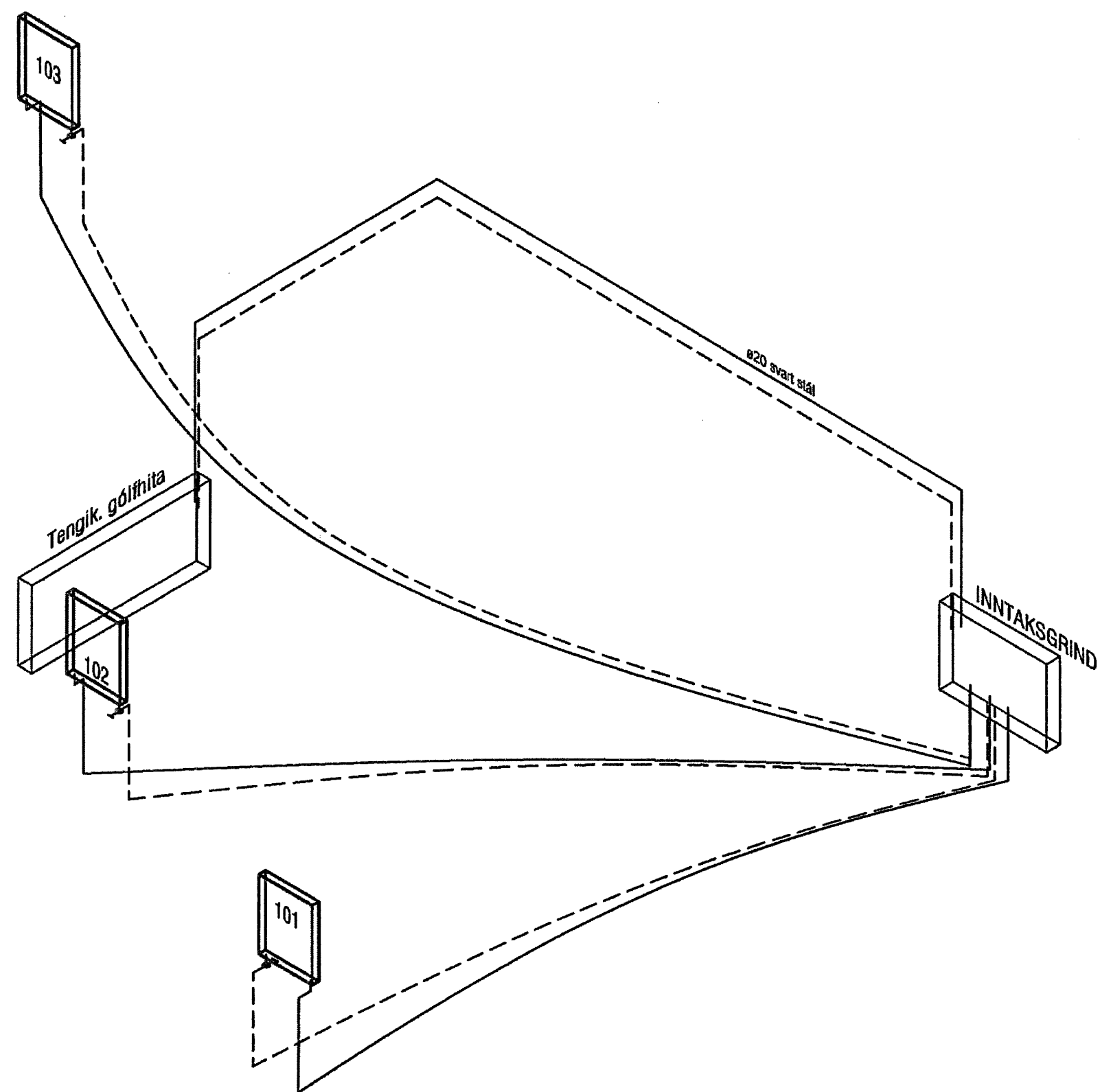
Rúmmynd neysluvatnslagna LAGNIR ERU ÚR P-PEX EDA ÁL-PEX RÖRUM SJÁ L-01
