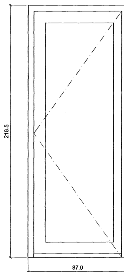
H2 1.stk útihurð, hægri hengd opnast út
