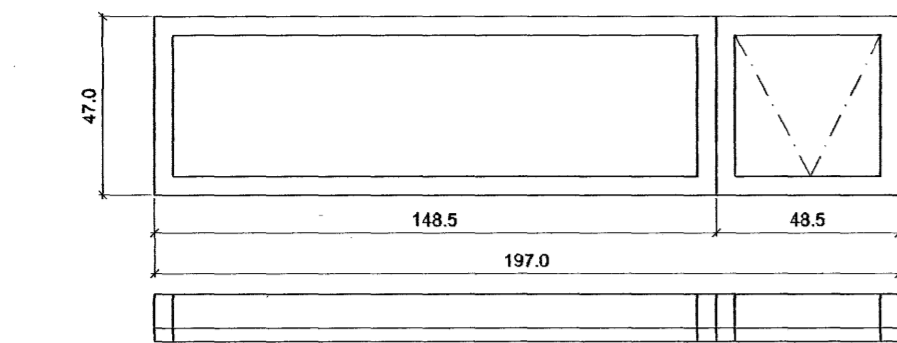
1 1stk, með opnanlegu fagi
