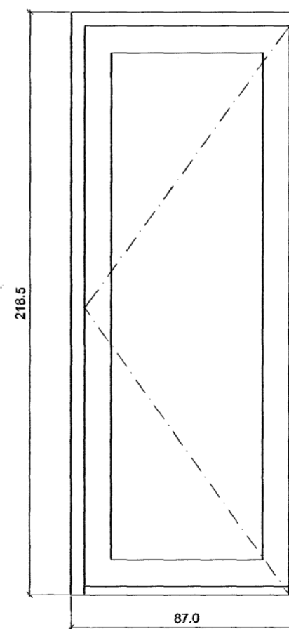
H4 1.stk útihurð, hægri hengd opnast út
