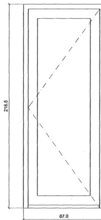
H3 1.stk útihurð, hægri hengd opnast út
