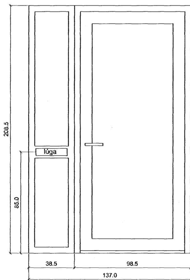
H1 1.stk útihurð, hægri hengd opnast inn
