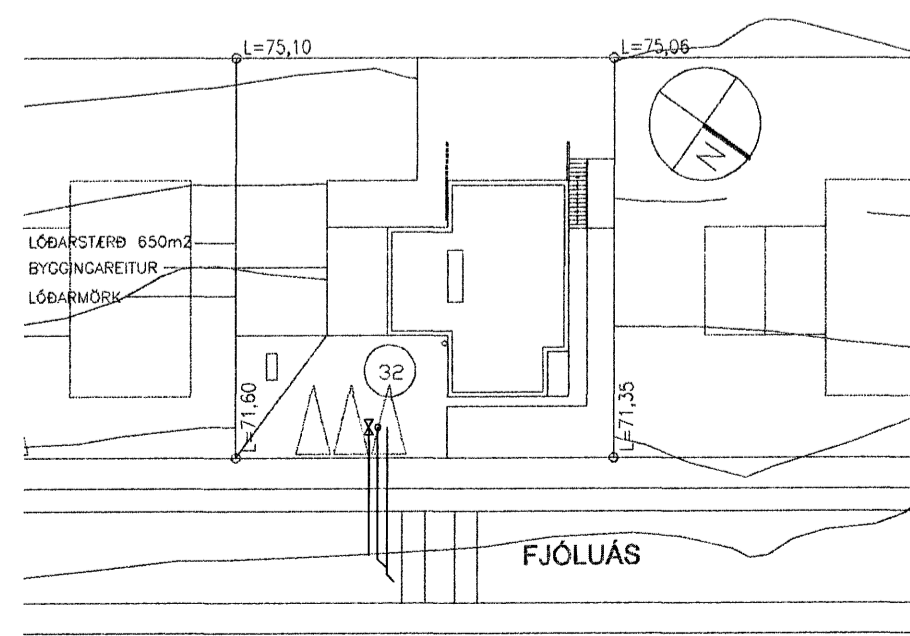
Afstöðumynd 1:500
