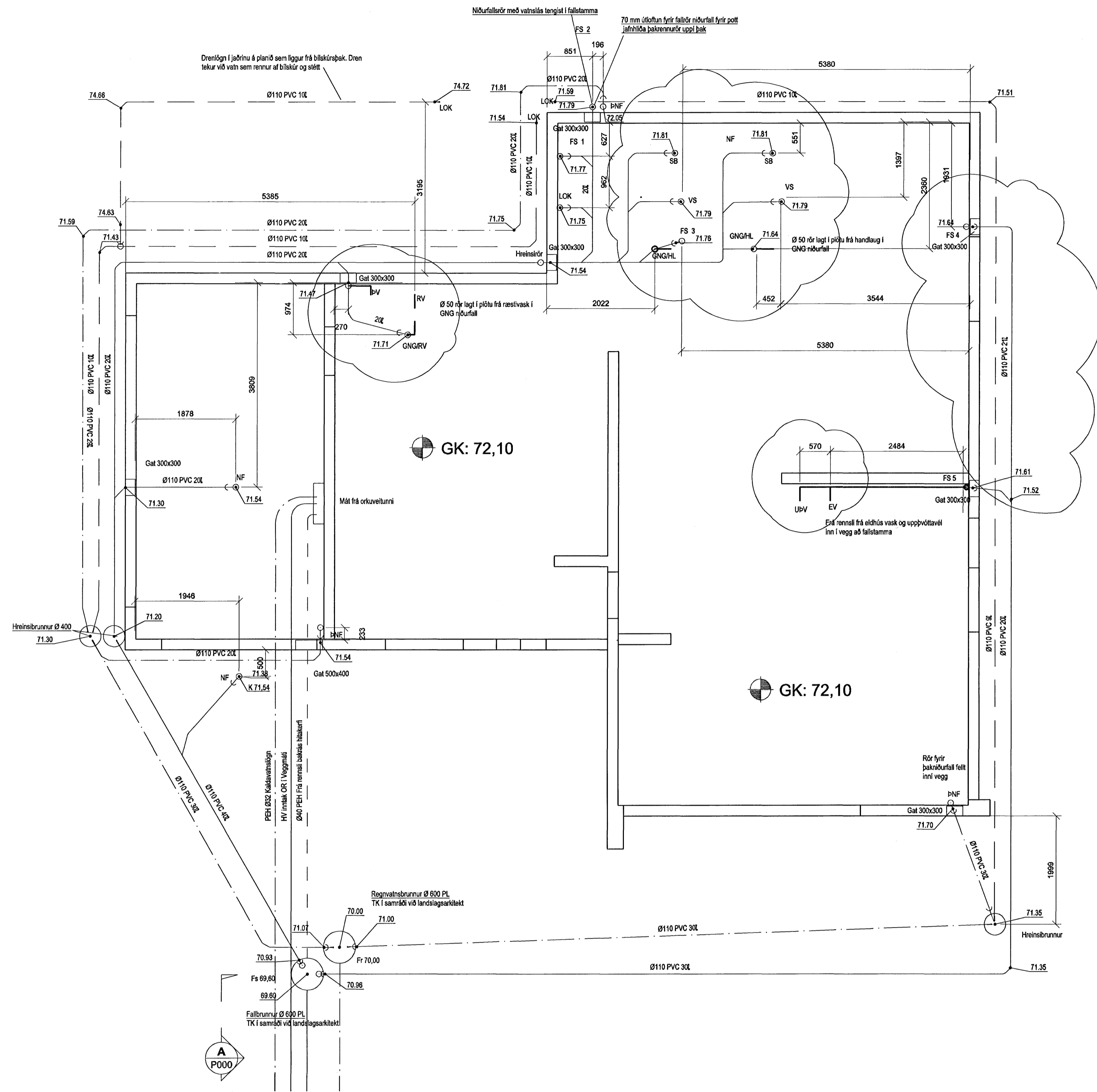
Afstöðumynd 1:500
