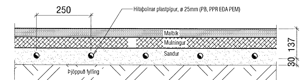
SNÍÐ Í SNJÓBRÆÐSLULAGNIR UNDIR MALBIKI, mkv. 1:10
