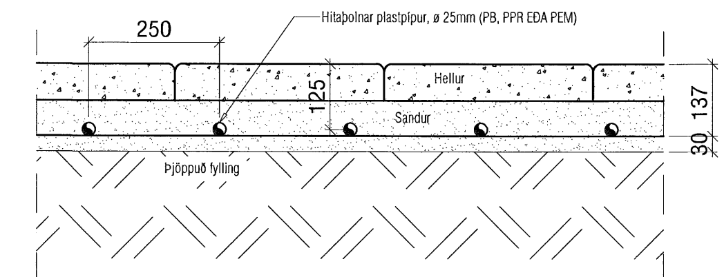
SNÍÐ Í SNJÓBRÆÐSLULAGNIR UNDIR HELLUM, mkv. 1:10
