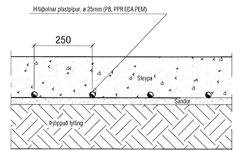
SNJÓBRÆÐSLULAGNIR Í STEYPTU PLANI, mkv. 1:10
