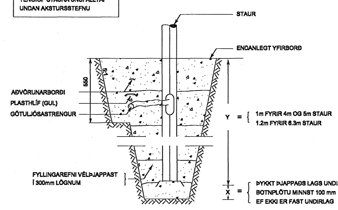
LJÓSASTAURAR 4/5/6,3 m
