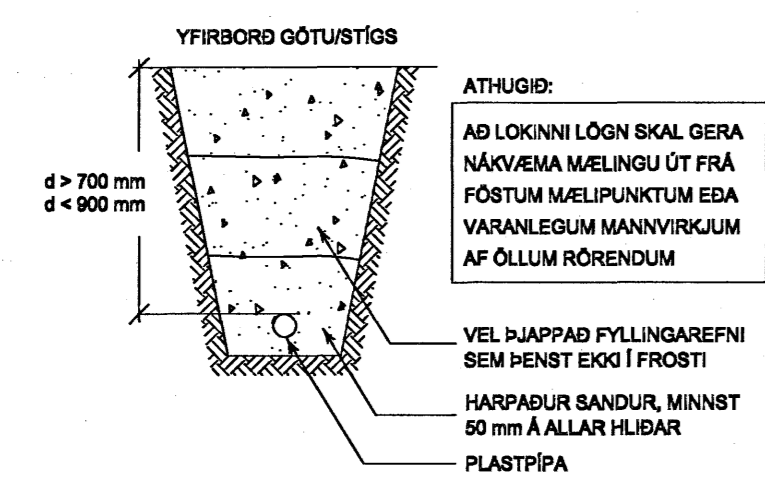
Jarðvinnusnið 1:20
